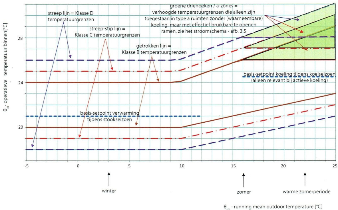
Figuur 1: Eisen (grenzen) voor de operationele temperatuur binnen, in relatie tot de running mean outdoor temperature (zie ISSO 74) [3], met aanvullend een weersafhankelijke setpointindicatie.
