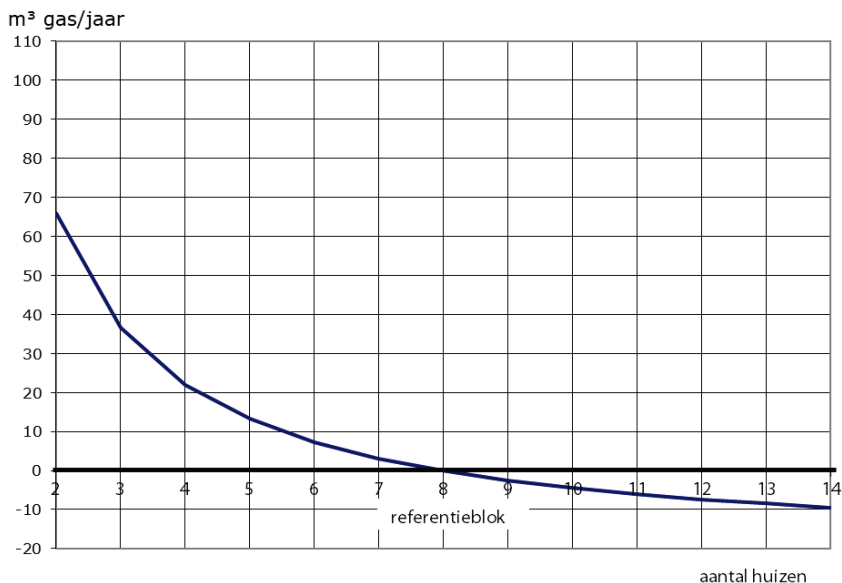
Afb. 4.2 De lengte van het bouwblok is van invloed op het gemiddelde energieverbruik voor ruimteverwarming per woning. Door de huidige goede warmte-isolatie is dit effect echter relatief beperkt. Door het verlengen van de bloklengte daalt het gemiddelde energieverbruik per woning; er komen immers meer tussenwoningen bij (met relatief weinig
