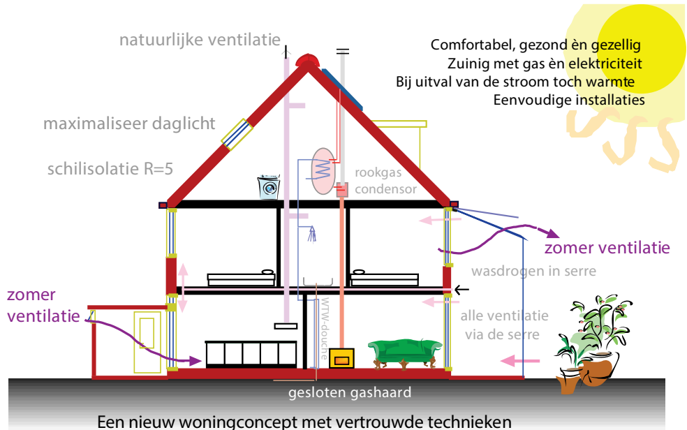
Afb. 3.10 Principe doorsnede van een zonnehaardwoning Wanneer in de serre was wordt gedroogd, deze eerst goed centrifugeren
