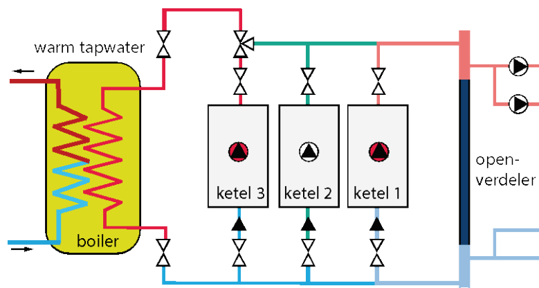
Afb. 7.30 Voorbeeld van een cascade-opstelling met voorkeurschakeling voor warmtapwater
