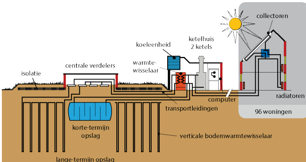
Afb. 7.34 Seizoenopslag voor zonnewarmte in het project Froukemaheerd in de Groningse wijk Beijum uit 1980. De opslag bestaat uit 15 km slangen aangebracht onder een centraal gelegen grasveldje. De opslag heeft een diameter van bijna 40 m en een diepte van 20 m en is aan de bovenzijde geïsoleerd. De 96 woningen zijn voorzien van totaal 2350 m 2 zonnecollectoren. Het verwarmingssysteem in de woningen bestaat uit lage temperatuur radiatoren. Er is een centrale bijstook met gasketels. Uit metingen blijkt dat de bijdrage van de zonne-energie aan de totale warmtevraag voor ruimte- en tapwaterverwarming ongeveer 65% bedraagt. De gemiddelde temperatuur van de bodem in de opslag varieert van circa 30 °C rond februari tot bijna 50 °C rond oktober. Het totale systeem functioneert nog steeds zonder bijzondere klachten. In de loop van de jaren zijn wel enige wijzigingen aangebracht en reparaties verricht [173]. In 2009 is het installatiesysteem gerenoveerd en aangepast [181]. Zo zijn er o.a. efficiëntere zonnecollectoren aangebracht zodat de collectoroppervlakte kleiner kon zijn en er ruimte vrij kwam om PV-panelen te plaatsen. De gewonnen warmte wordt nu (in tegenstelling tot voor de renovatie) direct in de desbetreffende woning voor tapwater gebruikt. Een overschot wordt per woonblok verzameld en voor ruimteverwarming gebruikt. Alleen als daarna nog warmte over is, wordt deze centraal opgeslagen. (Bron: Ontwerp: Architecten- en Ingenieursbureau Kristinsson i.s.m. Bredero Energy Systems; renovatie: BAM Techniek i.s.m. Nefit, Opdrachtgever: corporatie De Huismeesters)
