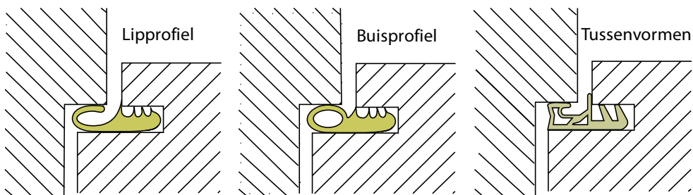
Afb. 5.30 Lipprofiel, Buisprofiel en Tussenvormen
