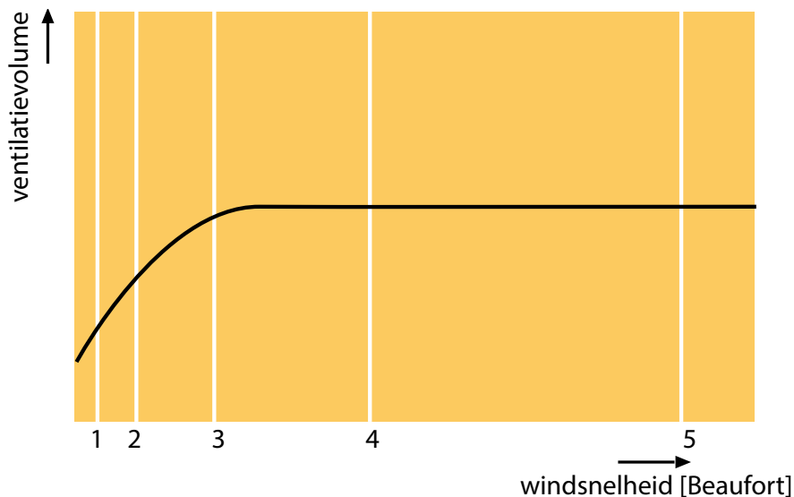
Afb. 6.10 Principe zelfregelend mechanisch ventilatierooster
