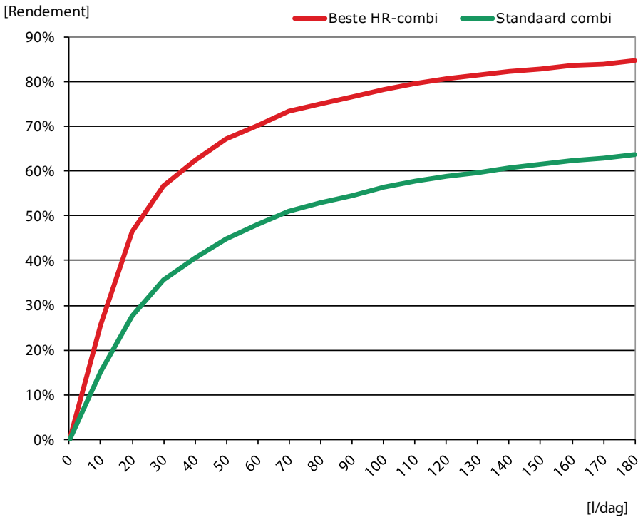
Afb. 9.9 Het gebruiksrendement is afhankelijk van de vraag. Het gebruik van een huishouden ligt tussen 60 en 180 liter per dag; per persoon gebruikt men globaal 40 liter heetwater per dag
