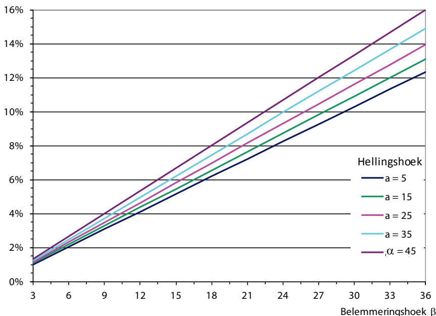
Afb. 10.5 Grafiek voor een indicatie van het effect van beschaduwing van zuidgerichte PV-panelen. Op de verticale as percentages (%) voor de vermindering van de opbrengst, op de horizontale de belemmeringshoek ( \beta ) in graden. De lijnen gelden voor PV-panelen onder verschillende hellingshoek ( a ), van 5° t/m 45°. (Bron: Grafiek afgeleid uit formule in [230])
