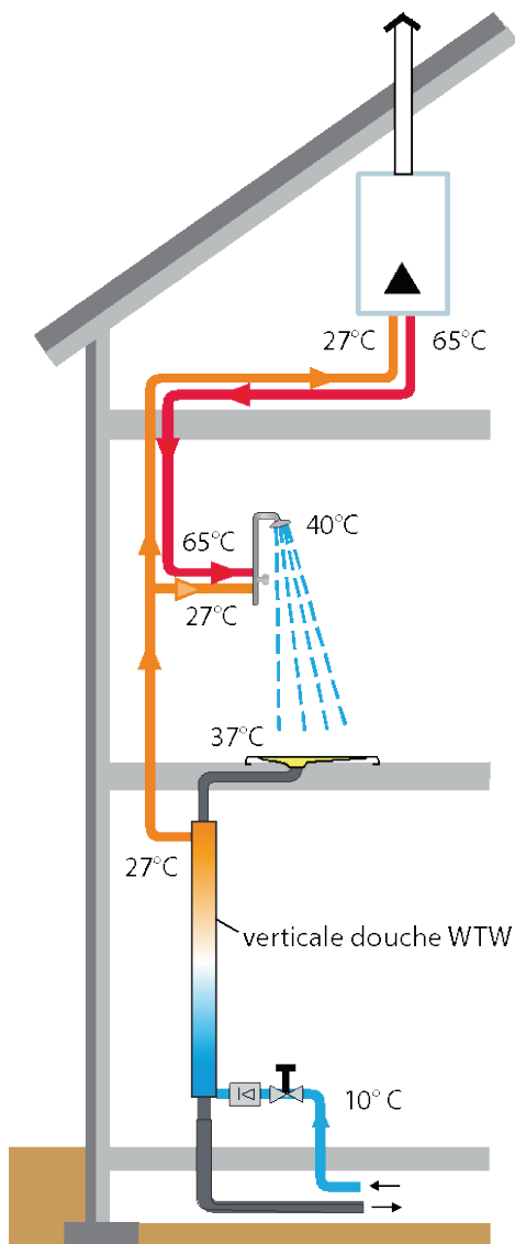
Afb. 9.4 Werkingsprincipe van de verticale douche(water)-WTW (warmteterugwinning); de douche-WTW bevindt zich op de begane grond. (Bron: Techna Duurzaam)
