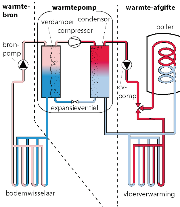
Afb. 7.21 Het principe van de warmtepomp
