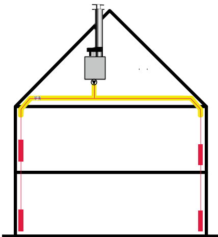
Afb. 7.14 Het isoleren van de CV-leidingen op de geïsoleerde zolder van de referentie tussenwoning bespaart zo'n 50 m 3 aardgas per jaar als de zolder niet verwarmd wordt
