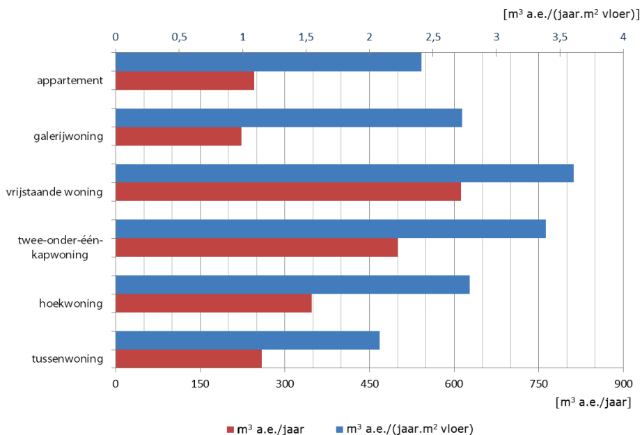
Afb. 4.1 De verschillen in het totale energieverbruik voor ruimteverwarming (gas + elektriciteit) plus elektriciteitsverbruik voor de ventilatie (in m^3 aardgasequivalent per jaar) van de RVO-referentiewoningen (met pakket 1, zie paragraaf 3.4) met een EPC van circa 0,4 en voorzien van ventilatiesysteem D3 (gebalanceerde ventilatie met CO_2 -sturing op de afvoer). Het energieverbruik voor verwarming en ventilatie hangt af van grootte en compactheid van het woningtype. Om alleen het effect van compactheid te laten zien, is ook het energieverbruik per vierkante meter gebruiksoppervlak gegeven
