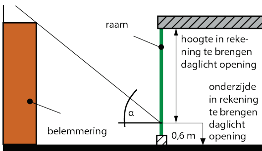
Afb. 4.21 De bepaling van de belemmeringshoek \alpha van belemmeringen binnen de perceelgrens. Alleen belemmeringen binnen een horizontale kijkhoek van 60^\circ tellen mee.
