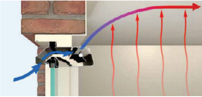
Afb. 6.11 Ventilatiooster waarbij door de vorm van het rooster de binnenkomende luchtstroom langs het plafond wordt geleid (door het Coanda-effect). In het stookseizoen wordt zo de ventilatielucht van buiten eerst gemengd (en opgewarmd) met binnenlucht. Dit verkleint de kans op koudeval en zorgt dus voor een comfortabeler binnenklimaat. (Bron: Alusta Natuurlijke Ventilatietechniek)
