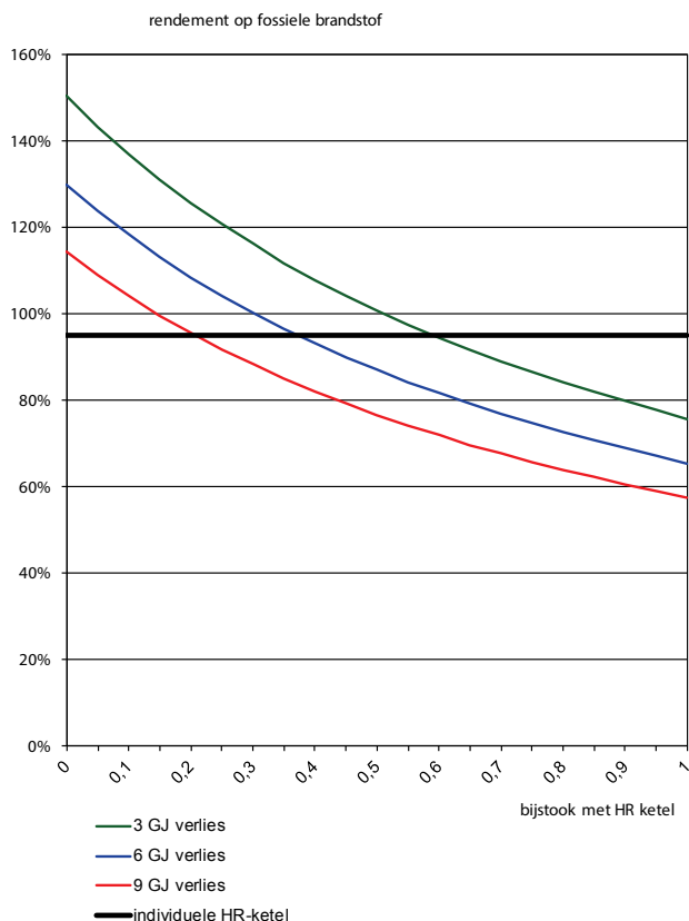
Afb. 7.36 Rendement op primaire energie van een collectief systeem afhankelijk van het percentage bijstook en het verlies van het distributiesysteem. 3 GJ verlies is alleen haalbaar bij blokverwarming, 9 GJ of meer is gebruikelijk bij warmtelevering. Uitgangspunten: rendement WKK 36% elektrisch, 50% warmte; rendement bijstook (HR-ketel op 75°C) 90%.); de warmtevraag (zonder bovenstaande verliezen) van de woning bedraagt 16 GJ inclusief tapwater. Rendement van de centrale opwekking die vermeden wordt is 50% conform NEN 7120 (zie in norm bij geëxporteerde energie). Alle rendementen op bovenwaarde. (Bron: BOOM-SI)
