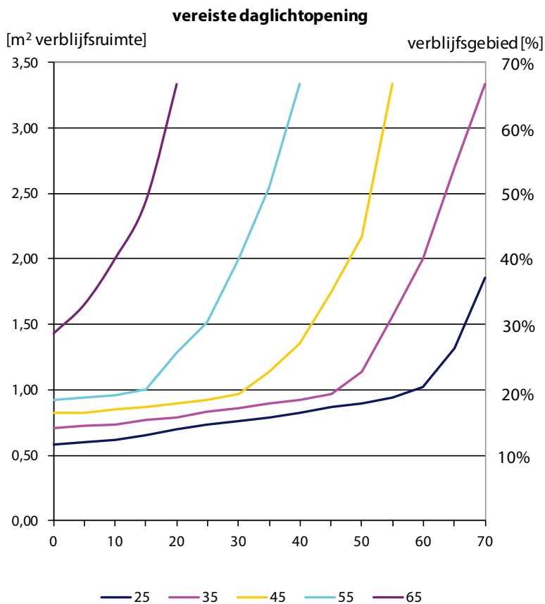
Afb. 4.24 Werkelijke daglichtopeningen om te voldoen aan de vereiste equivalente daglichtopening voor een verblijfsruimte (links m 2 ) en verblijfsgebied (rechts % vloeroppervlak) bij verschillende belemmeringshoeken \alpha en overstekhoeken \beta . Berekend volgens NEN 2057 [82].
