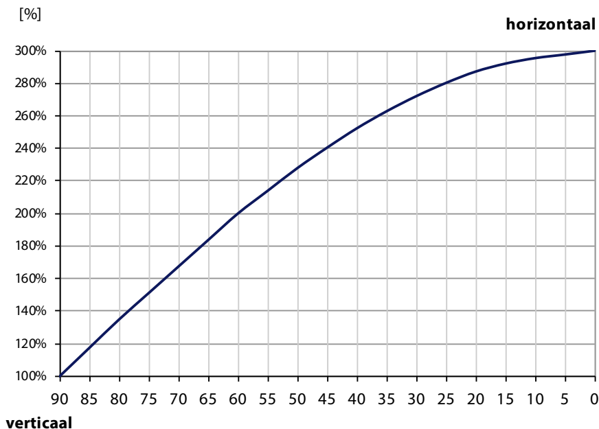
Afb. 4.26 De werkelijke lichtopbrengst ten opzichte van een verticaal raam (helling 90°) bij verschillende hellingshoeken volgens de CIE-hemel [Tabellarium Bouwfysica TU-Delft]. Door een horizontaal (dak)raam komt dus 3x zoveel daglicht binnen.
