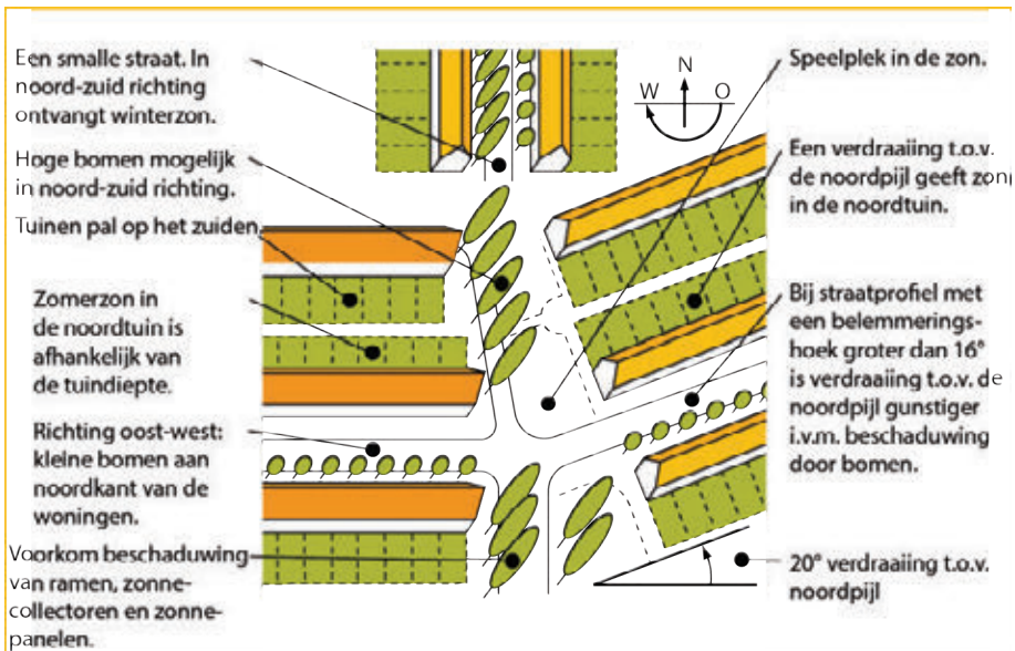
Afb. 4.8 Diverse ontwerpkeuzes voor de verkaveling gelet op bezonning [78]
