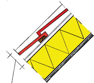
Afb. B.1-7 Warmteweerstand voor veel voorkomende luchtlagen in een spouwmuur en in een hellend dak met dakpannen, volgens NEN 1068 [107]. Bij toepassing van een reflecterende folie op de isolatie aan de spouwzijde bedraagt de R_{cav} 0,57 i.p.v. 0,18. Let op dat het effect van de folie niet dubbel geteld wordt: èn bij het isolatiemateriaal (inclusief folie) èn bij de spouw
