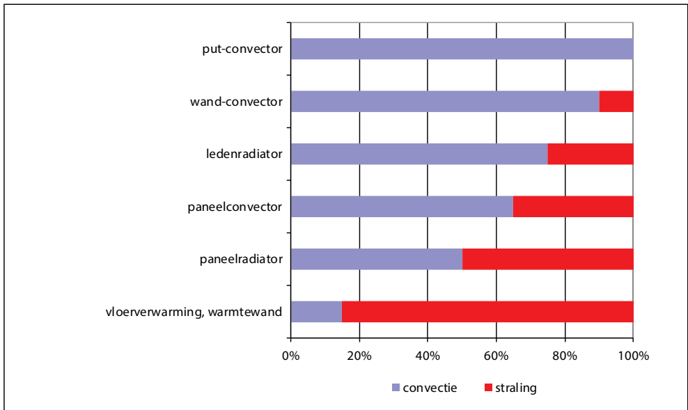
Afb. 7.2 Aandeel straling en convectie van de verschillende typen water-CV verwarmingselementen. Om eenzelfde gevoelstemperatuur te realiseren kan, bij een groter stralingsaandeel, de gemiddelde luchttemperatuur in een vertrek lager zijn. Dit werkt energiebesparend: Zowel de transmissie- als de ventilatieverliezen nemen af. Gebruik bij voorkeur een relatief lage watertemperatuur in combinatie met een relatief groot verwarmend oppervlak
