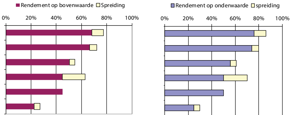
Afb. 9.9 Het gebruiksrendement is afhankelijk van de vraag. Het gebruik van een huishouden ligt tussen 60 en 180 liter per dag; per persoon gebruikt men globaal 40 liter heetwater per dag
