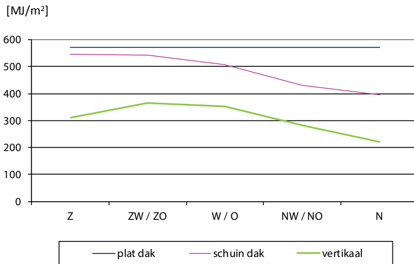
Afb. 4.14 De grafiek geeft de zonnestraling op een vierkante meter glas in de maand juni
