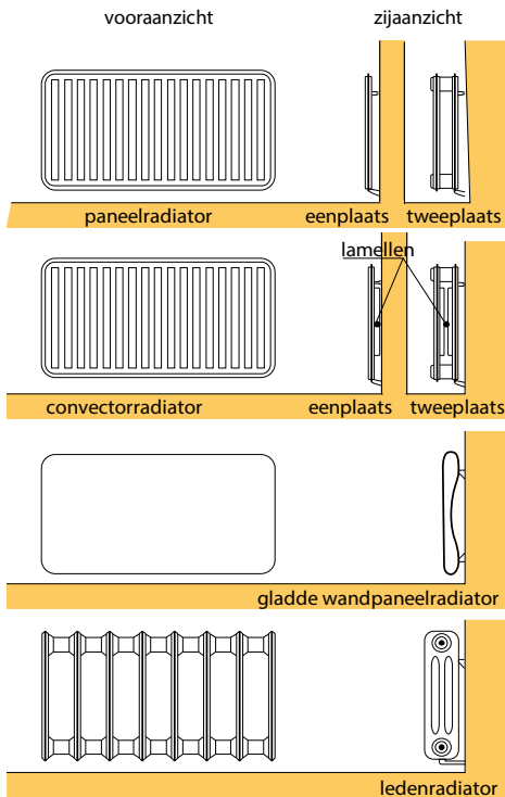
Afb. 7.3 De verschillende typen radiatoren
