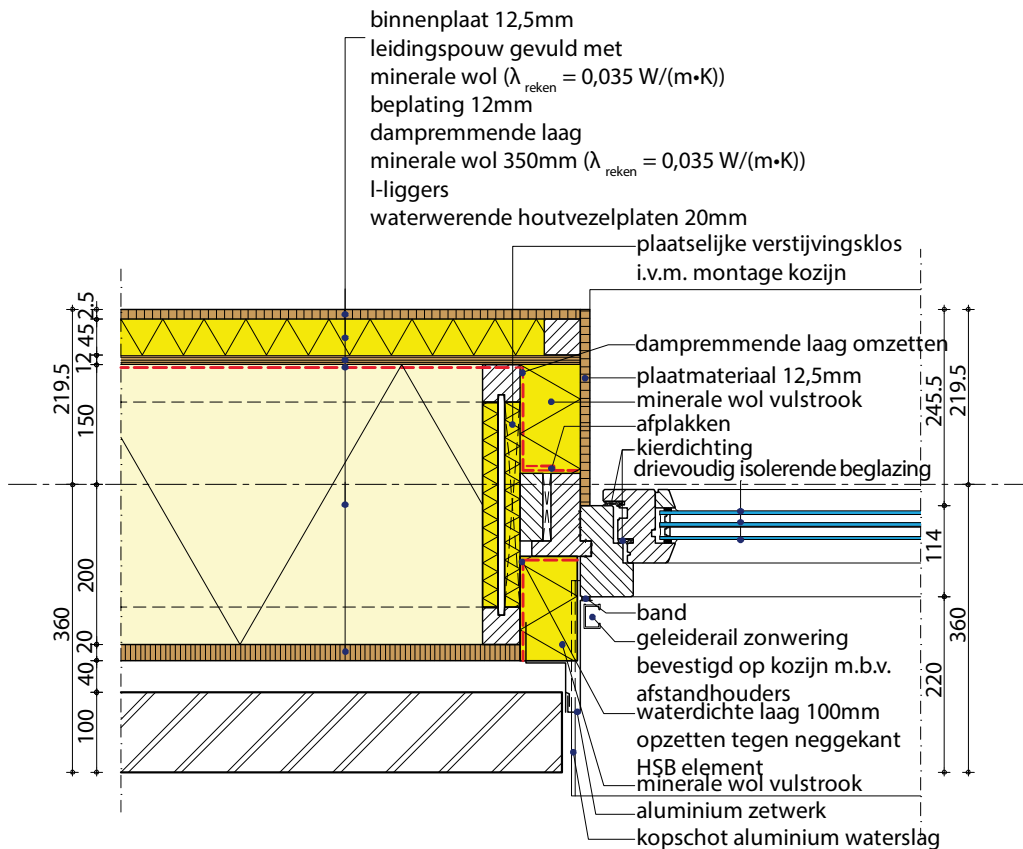
Afb. 3.9 Horizontale doorsnede. Voorbeeld van de aansluiting kozijn met het gesloten deel van de langsgevel in houtskeletbouw. Aan de binnenzijde (nog binnen de dampremmende laag) is een kleine spouw (gevuld met minerale wol) opgenomen waarin leidingen kunnen worden opgenomen. Deze spouw voorkomt dat de dampremmende laag onderbroken wordt waardoor vocht in de constructie kan komen en de luchtdichtheid afneemt. Bron [63].
