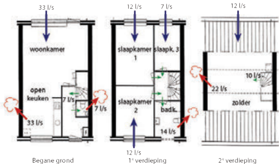
Afb. 6.3 Voorbeeld van de ventilatiestromen in de referentietussenwoning (van RVO) die (in dit voorbeeld) voorzien is van ventilatiesysteem C: natuurlijke toevoer van buitenlucht via ventilatieroosters in de gevels (blauwe pijlen) en mechanische afvoer (rode pijlen) via een centrale ventilatie-unit
