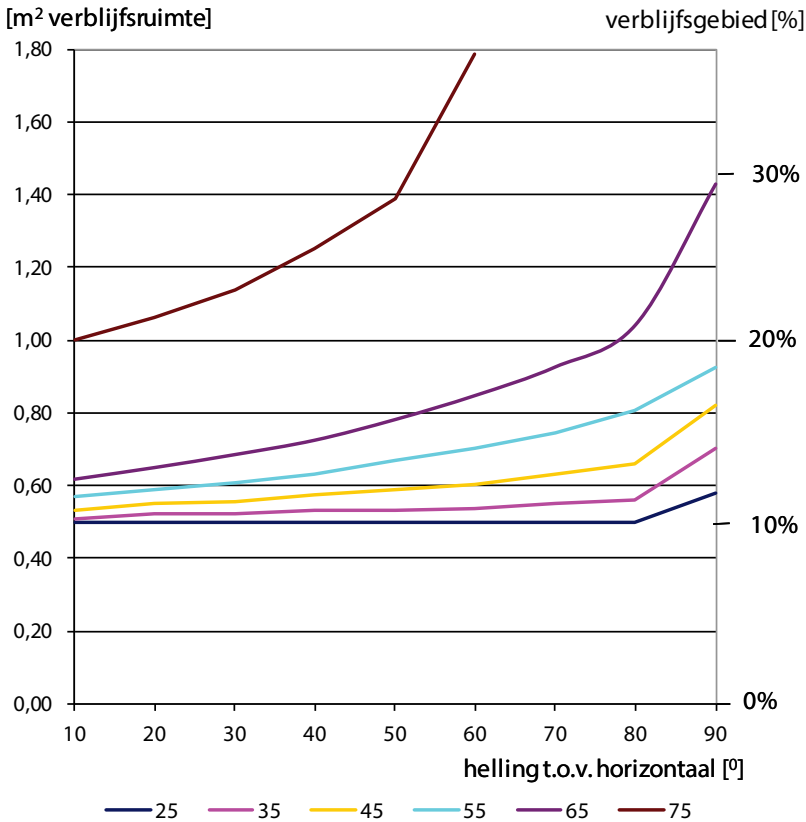
Afb. 4.25 Werkelijke daglichtopening om te voldoen aan de vereiste equivalente daglichtopening voor een dakraam voor een verbljfsruimte (links m 2 ) en verbljfsgebied (rechts %) bij verschillende belemmeringshoeken \alpha . De overstekhoek \beta is in alle gevallen 0. In alle gevallen ligt het hart van het raam op een hoogte van 1,7 meter. Berekend volgens NEN 2057 [82].
