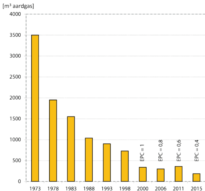
Afb. 1.10 Jaarlijks energieverbruik in m³ aardgas voor ruimteverwarming (excl. elektriciteit voor CV-pomp) van een gemiddelde nieuwbouwwrijtjeswoning gespecificeerd naar bouwjaar. Het gaat hierbij om berekende waarden. De waarden voor 2011 en 2015 zijn berekend met NEN 7120 (EPG). (Bron: [13] en referentiewoningen van RVO vanaf 1993)
