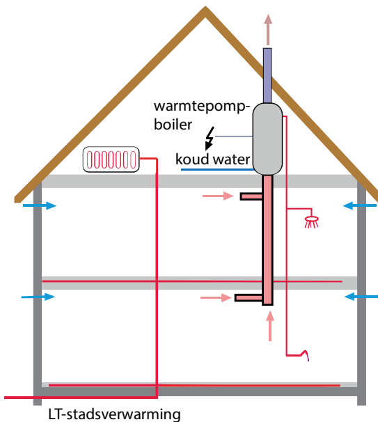
Afb. 9.23 Een schema van een warmtepompboiler
