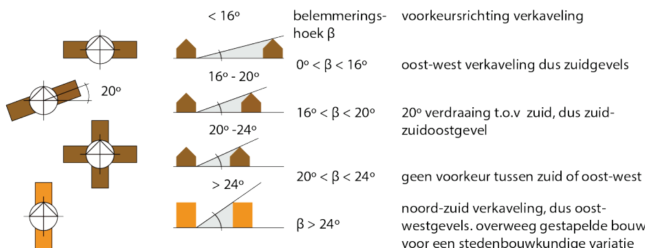
Afb. 4.4 Verkavelingsrichting voor eengezinswoningen bij een bepaalde belemmeringshoek
