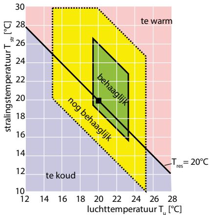
Afb. B.1-2 Samenhang tussen luchttemperatuur en stralingstemperatuur bij een relatieve vochtigheid van 0,1 tot 0,2 m/s. Uit de grafiek blijkt dat een T_{res} van 20 °C nog geen garantie hoeft te zijn voor een behaaglijk binnenklimaat. (Bron: [244])
