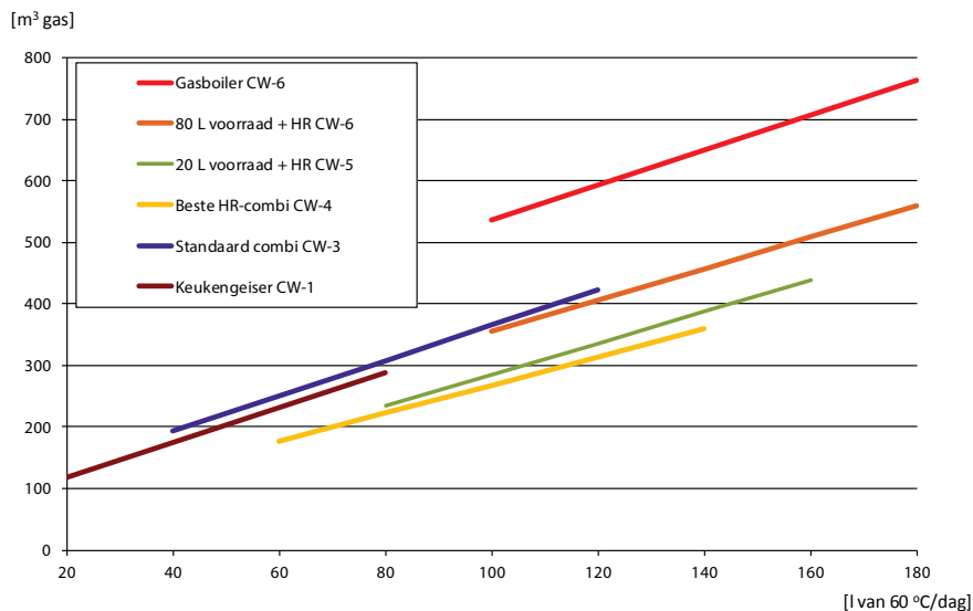
Afb. 9.8 Het gasverbruik per jaar (op de verticale as) van verschillende toestellen afhankelijk van de vraag aan het toestel en het geboden comfort. Een hogere CW-klasse roept een grotere vraag op. Door het toepassen van warmwaterbesparing, douche-WTW en zonneboilers, is er een dalende trend
