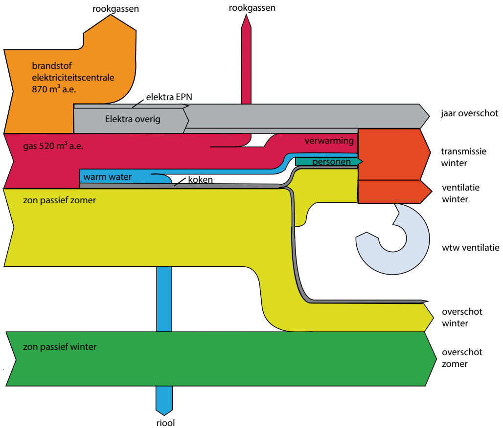
Afb. 1.14 Een indicatie van de energiestromen in de referentie tussenwoning (voorzien van pakket 1, zie paragraaf 3.4) voor een gemiddeld huishouden op basis van EPC-berekening en statistische gegevens (met name voor elektriciteitsverbruik voor huishoudelijke apparaten) in m³ aardgasequivalent per jaar. Een dergelijk stromendiagram wordt wel een Sankey-diagram genoemd
