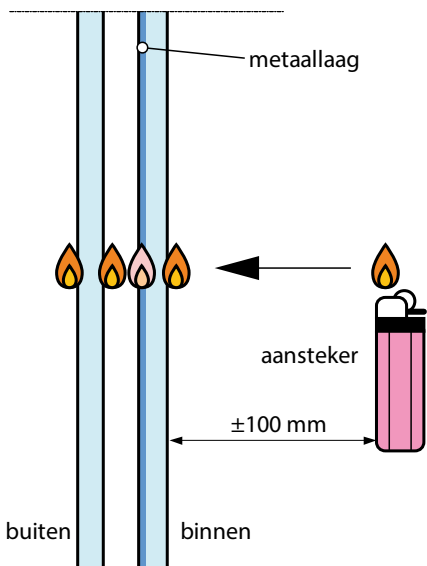
Afb. 5.34 Trucje ter controle van de juiste plaatsing van goed-isolerend glas (met metaallaag): Houd aan de woningzijde van het glas, op \pm 0,1 m afstand hiervan, een brandende aansteker. Naar buiten kijkend, zie je dan (bij HR ++ - glas) vier vlammetjes reflecteren. Het tweede vlammetje behoort een afwijkende kleur, meestal blauw/rose, te hebben omdat in dit voorbeeld de metaallaag op de binnenste glaslaag aan de spouwzijde is aangebracht.
