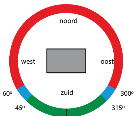
Afb. 10.4 Richtlijnen voor helling en oriëntatie zonnepanelen. Zie het Zonneinstralingsdiagram in Bijlage 7 voor meer gedetailleerde informatie.
