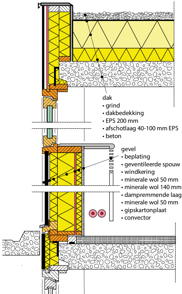
Afb. 5.16 Doorsnede van één van de gevels van het project 'Urban Villa' in Amstelveen, een voorloper van de passiefhuizen en een vervolg op de Minimum Energie Woningen uit 1983. Het isolatiepakket bestaat uit totaal 240 mm minerale wol. In de isolatie ligt de dampremmende laag waardoor deze goed beschermd is. Het stijl- en regelwerk ligt niet in één vlak zodat slechts op de plek waar ze elkaar kruisen de constructie uit alleen hout zonder isolatie bestaat. Dit beperkt het warmteverlies. (Bron: Architect: Atelier Z - Zavrel Architecten; Ontwikkeling: BAM Vastgoedbeheer en RABO Vastgoed; Onderzoek en advies: Damen Consultants, TU-Delft en DWA. Realisatie: 1995)
