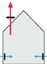
Afb. 6.21 Principe gebalanceerde ventilatie met decentrale toevoer en centrale afvoer
