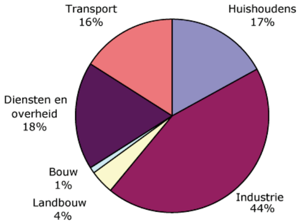
Afb. 1.5 Verdeling van het totale Nederlandse primaire energieverbruik naar sector in 2013; afgeleid uit cijfers van 2007 van ECN en [9]. Het totale verbruik in 2013 bedroeg circa 3219 PJ
