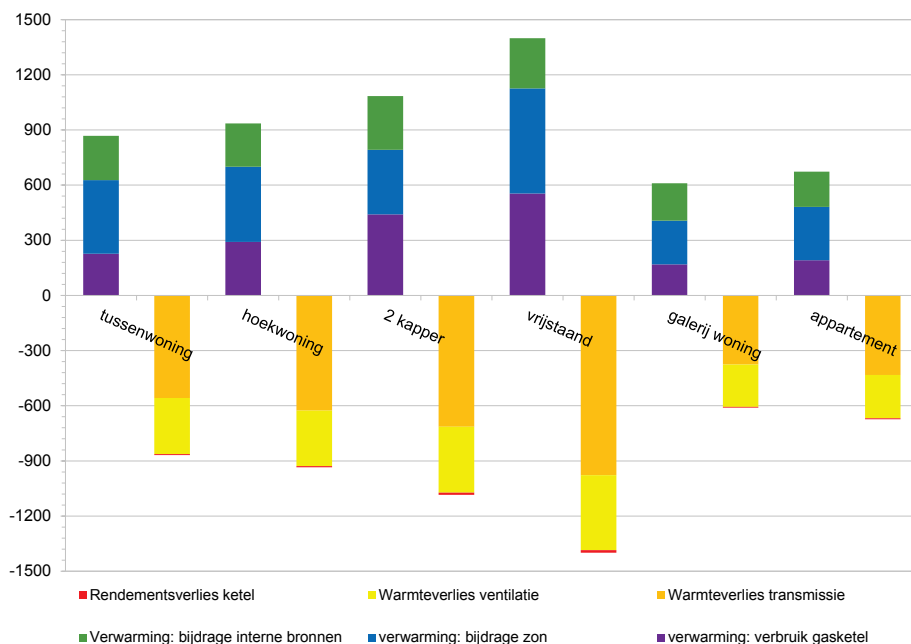
Afb. 1.13 De grafiek illustreert voor de zes RVO referentiewoningen met EPC van circa 0,4 (voorzien van pakket 1, zie paragraaf 3.4) de relevante warmtestromen voor ruimteverwarming (in m 3 aardgasequivalent)
