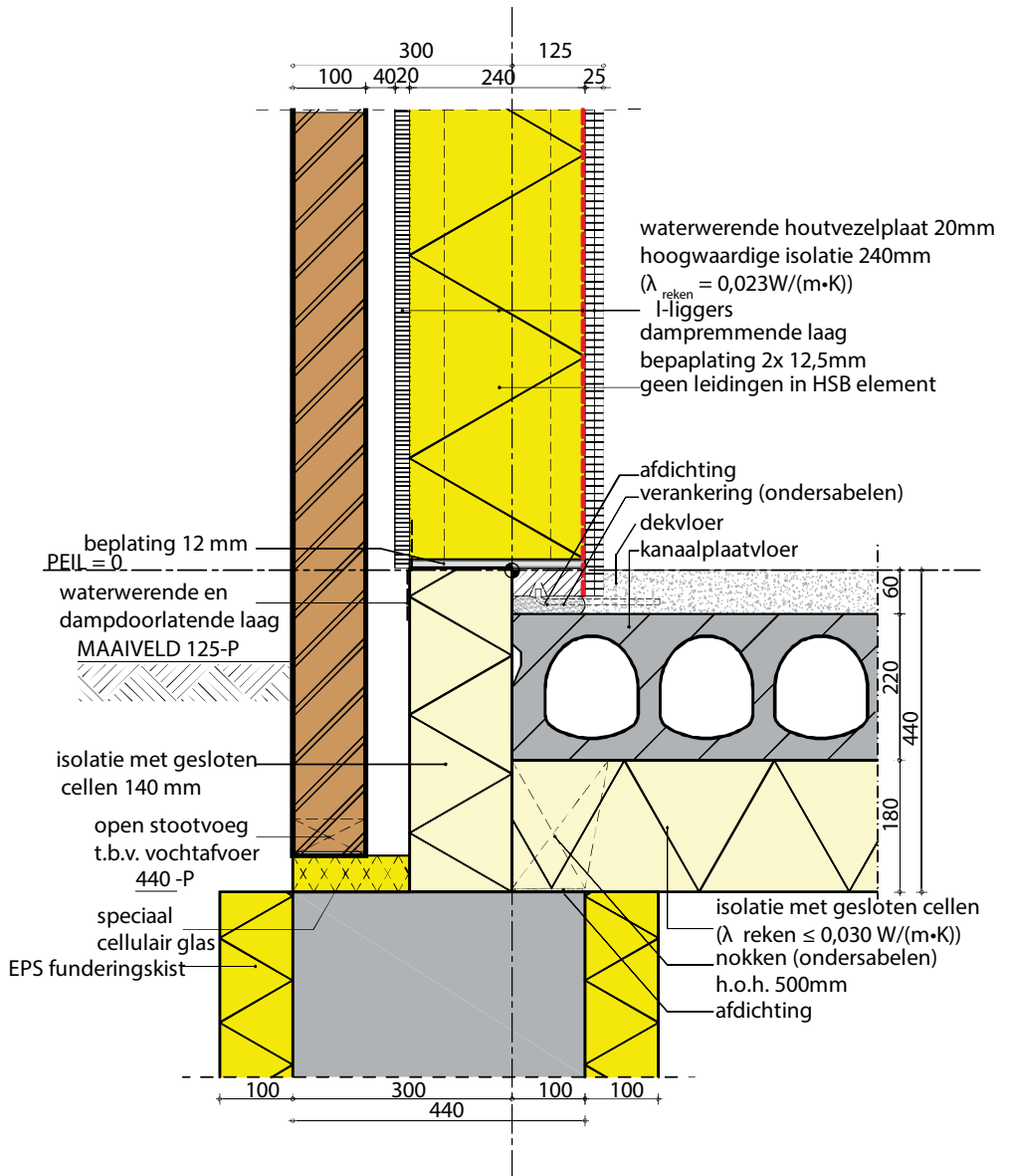
Afb. 3.8 Verticale doorsnede. Voorbeeld van de aansluiting fundering met langsevel in een Passiefhuis. In het binnenspouwblad is een isolatiemateriaal gebruikt met een \lambda -waarde van 0,23 (bijv. PIR-schuim); als er minerale wol met een \lambda -waarde van 0,035 wordt gebruikt, neemt de isolatiedikte toe van 240 mm naar ca. 340 mm. Om de koudebrug van de constructie in het binnenblad te beperken is een houten I-ligger gebruikt. Het gemetselde buitenspouwblad staat op cellulair glas, eveneens om de koudebrug via de fundering te minimaliseren. Bron [63].
