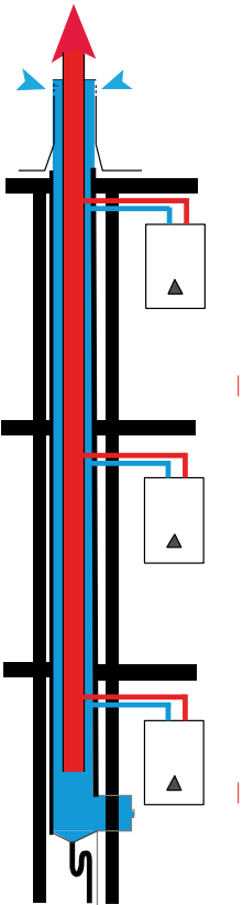
Afb. 7.17 Een voorbeeld van een CLV-systeem
