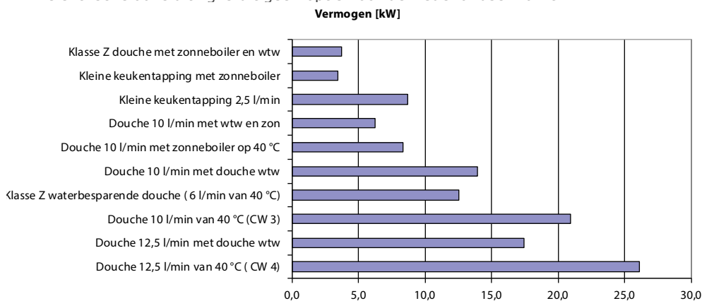
Afb. 9.11 Benodigd vermogen van een doorstroomtoestel onder verschillende condities.
