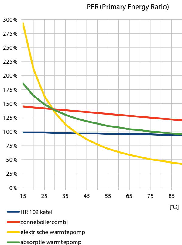
Afb. 7.25 Indicatie van de PER van een elektrische en gasgestookte warmtepomp, zonneboilercombi en van een HR107-ketel, afgezet tegen het temperatuurverschil dat de warmtepomp moet overbruggen tussen de bron en het afgiftesysteem. Voor de HR-ketel en de zonneboilercombi is de aanvoertemperatuur van de CV-installatie genomen. De investering voor de beide warmtepompen en de zonneboilercombi zijn globaal hetzelfde. Duidelijk blijkt hoe sterk de PER van warmtepompen afhangt van het genoemde temperatuurverschil
