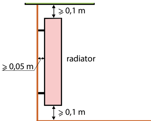
Afb. 7.4 Plaats radiatoren (en wandconvectoren) met voldoende afstand tot vloer, gevel en vensterbank. Dit in verband met schoonmaak en de benodigde convectie-luchtstroming. Zorg er voor dat (in het stookseizoen) de opgaande warme luchtstroom van de radiatoren niet achter eventuele (rol)gordijnen of jaloezieën kan terechtkomen. Stem de detaillering van de vensterbank en de plaatsing van gordijnen ed. hierop af. De vensterbank mag ook de warmte-afgifte aan de kamer niet belemmeren. Plaats in de badkamer de radiator op een hoogte van minimaal 0,6 meter vanaf de vloer om roesten te voorkomen. Kies desnoods voor een verzinkte radiator in de badkamer
