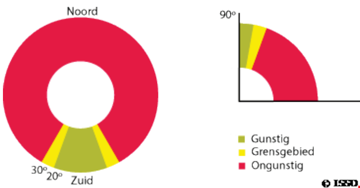
Afb. 4.15 Optimale oriëntatie en hellingshoek voor ramen. Een hellingshoek van 90° heeft de voorkeur om te hoge temperaturen in de zomer te voorkomen. Bovendien is de nachtelijke uitstraling bij verticale ramen het geringst. Als er houten kozijnen gebruikt worden, is het uit het oogpunt van onderhoud sowieso ongewenst om ze onder een hellingshoek aan te brengen
