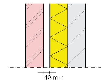
Afb. B.1-6 Warmte-overgangsweerstanden (= warmteweerstand) van de diverse luchtlagen grenzend aan een constructie. De waarden van R_{si} en R_{se} zijn sterk afhankelijk van de luchtsnelheid nabij de constructie; over het algemeen worden de in de afbeelding aangegeven vaste waarden gehanteerd. R in m^2 \cdot K/W . (Bron NEN 1068) [107]
