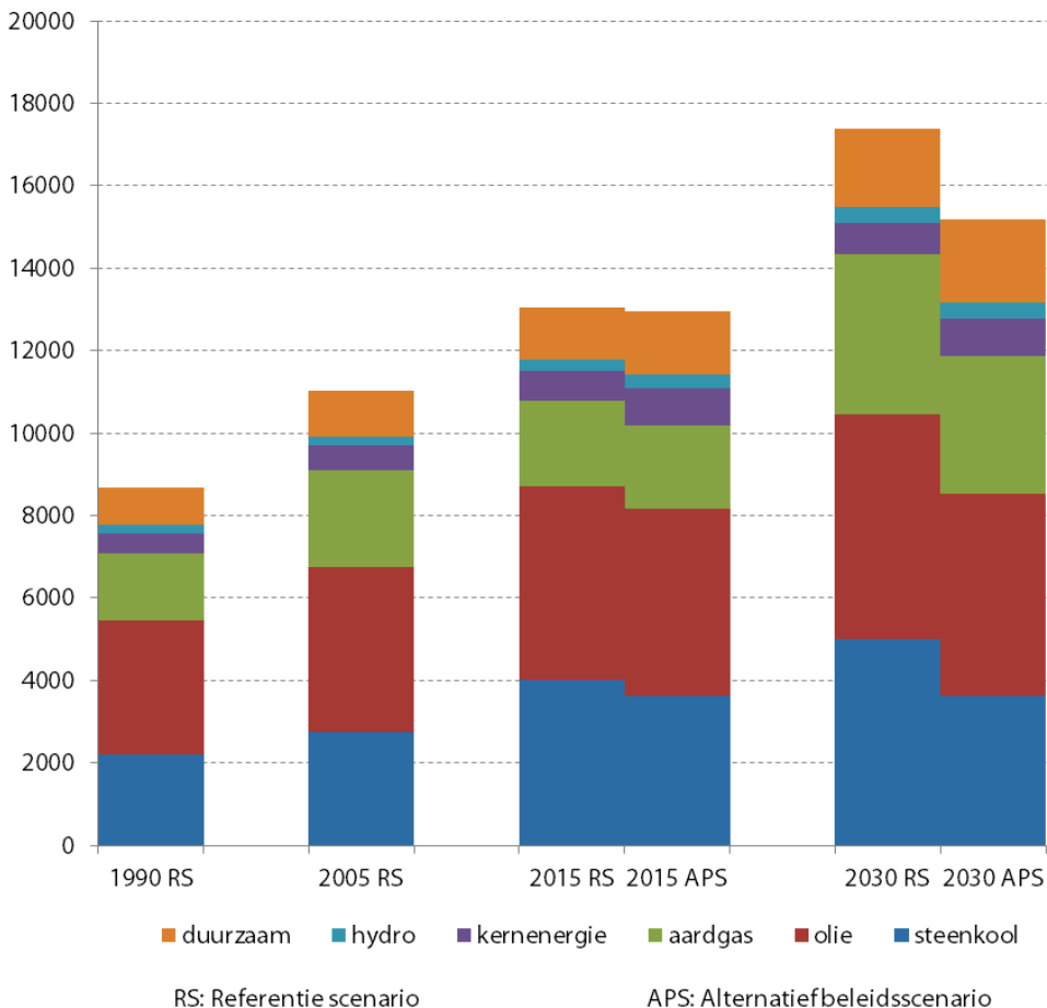
Afb. 1.4 De (mogelijke) ontwikkeling van het wereldenergieverbruik van 1990 tot 2030 volgens 2 scenario's: het referentiescenario (RS) volgens de huidige energiepolitiek en een alternatief scenario (AS) met verdergaande besparingsmaatregelen. Onder 'overige bronnen' vallen de verschillende duurzame bronnen zoals biobrandstoffen, wind en zon. (Bron: IEA [8])
