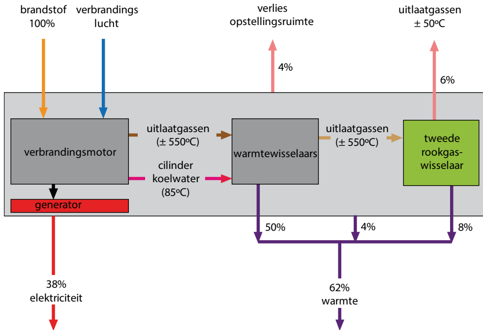
Afb. 7.28 Werkingsprincipe van een WKK-eenheid. Rendementen op onderwaarde
