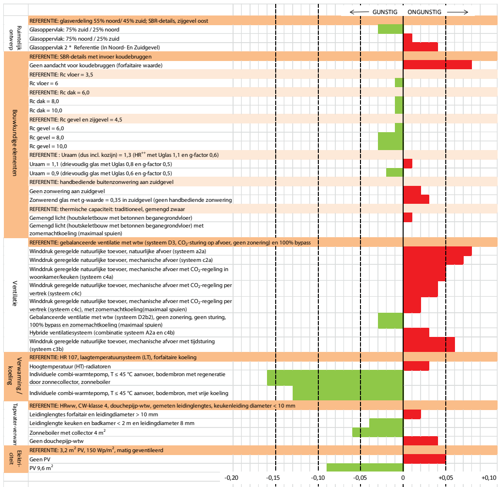
Afb. 3.2 Het effect van een aantal energiebesparende maatregelen op de EPC van de referentie twee-onder-een-kapwoning van RVO (voorzien van pakket 1 uit afb 3.3; EPC =
