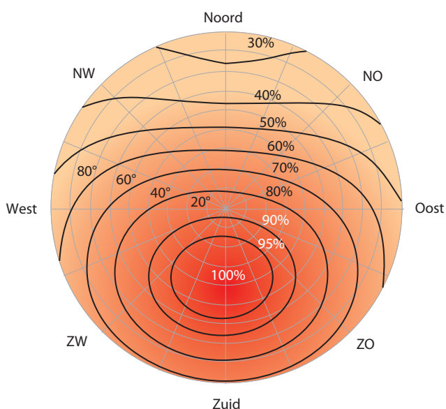
Afb. B.7-2 Zonne-instralingsdiagram
