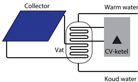
Afb. 9.18 De CV-zonneboiler. Het systeem is vergelijkbaar met een indirect gestookte boiler
