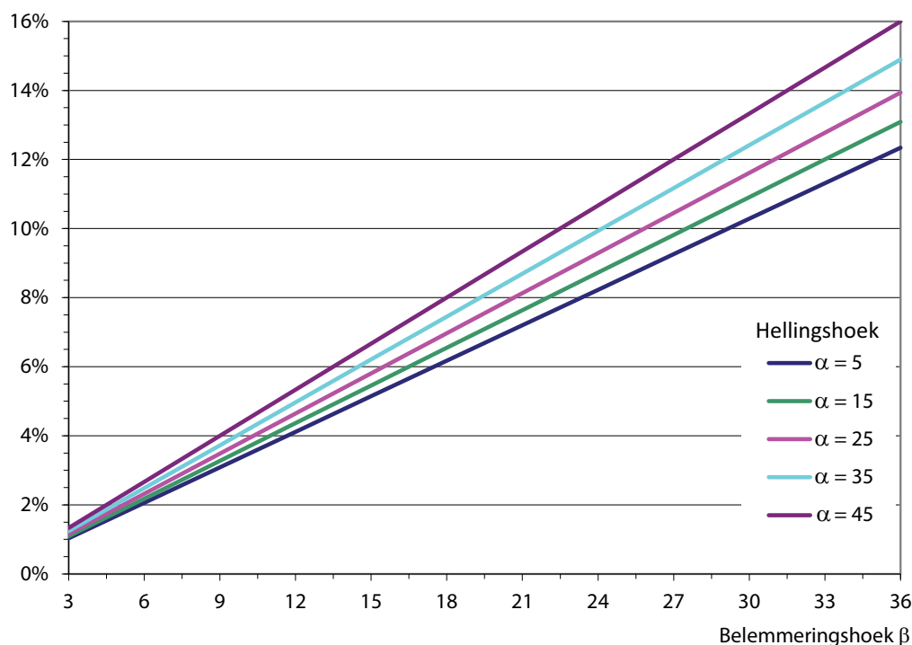
Afb. 10.5 Grafiek voor een indicatie van het effect van beschaduwing van zuidgerichte PV-panelen. Op de verticale as percentages (%) voor de vermindering van de opbrengst, op de horizontale de belemmeringshoek ( \beta ) in graden. De lijnen gelden voor PV-panelen onder verschillende hellingshoek ( \alpha ), van 5° t/m 45°. (Bron: Grafiek afgeleid uit formule in [230])
