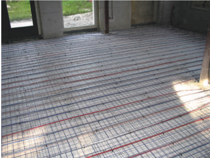
Afb. 8.2 Het afgiftesysteem voor vloerkoeling is hetzelfde als voor vloerverwarming. Een systeem met direct een isolatielaag er onder reageert veel sneller dan een systeem zonder die isolatie (zie ook paragraaf 7.2.3). Op de foto moet de dekvloer nog worden aangebracht
