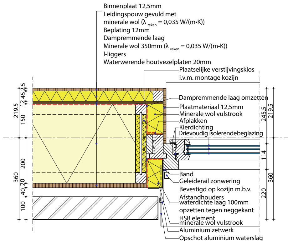
Afb. 3.9 Horizontale doorsnede. Voorbeeld van de aansluiting kozijn met het gesloten deel van de langsevel in houtskeletbouw. Aan de binnenzijde (nog binnen de dampremmende laag) is een kleine spouw (gevuld met minerale wol) opgenomen waarin leidingen kunnen worden opgenomen. Deze spouw voorkomt dat de dampremmende laag onderbroken wordt waardoor vocht in de constructie kan komen en de luchtdichtheid afneemt. Bron [63].
