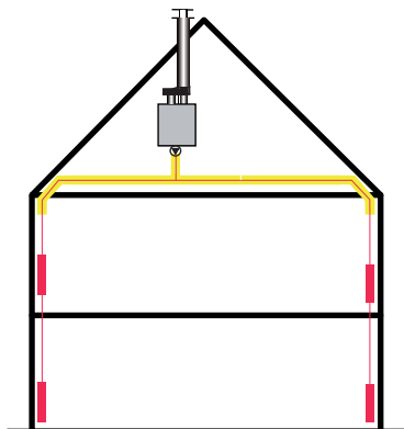
Afb. 7.14 Het isoleren van de CV-leidingen op de geïsoleerde zolder van de referentie tussenwoning bespaart zo'n 50 m 3 aardgas per jaar als de zolder niet verwarmd wordt
