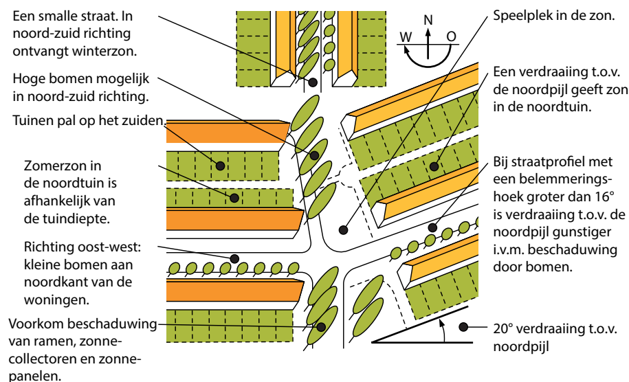
Afb. 4.8 Diverse ontwerpkeuzes voor de verkaveling gelet op bezonning [78]
