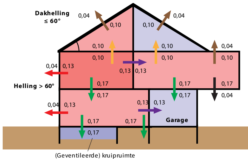
Afb. B.1-6 Warmte-overgangsweerstanden (= warmteweerstand) van de diverse luchtlagen grenzend aan een constructie. De waarden van R_{si} en R_{se} zijn sterk afhankelijk van de luchtsnelheid nabij de constructie; over het algemeen worden de in de afbeelding aangegeven vaste waarden gehanteerd. R in m^2 \cdot K/W . (Bron NEN 1068) [107].
