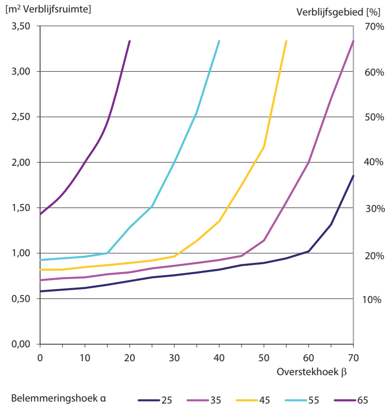
Afb. 4.24 Werkelijke daglichtopeningen om te voldoen aan de vereiste equivalente daglichtopening voor een verblifruimte (links m^2 ) en verblifgebied (rechts % vloeroppervlak) bij verschillende belemmeringshoeken \alpha en overstekhoeken \beta . Berekend volgens NEN 2057 [82].
