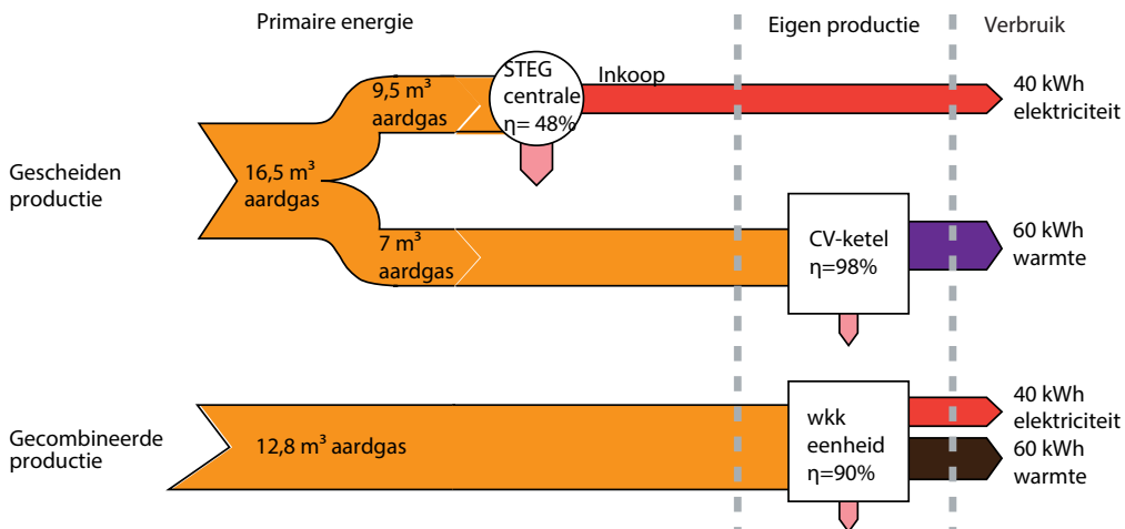
Afb. 7.27 Verskil in primair energieverbruik tussen een gescheiden en een gecombineerde productie van warmte en elektriciteit
