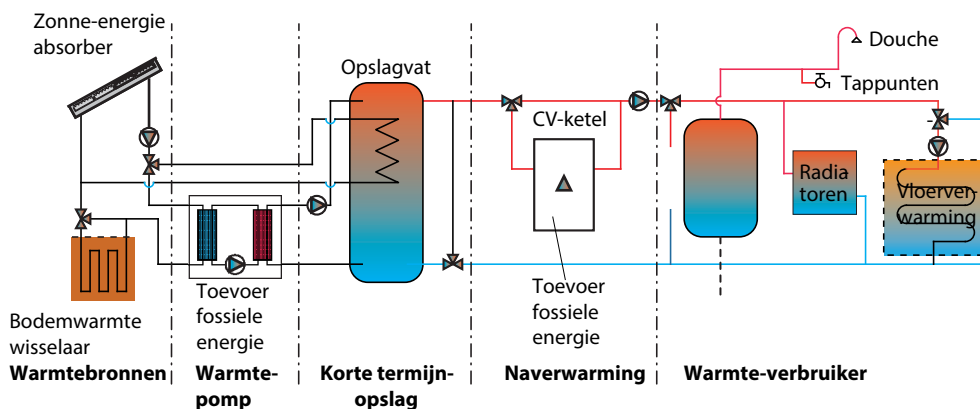
Afb. 7.26 Toepassing van warmtepomp in combinatie met andere apparatuur
