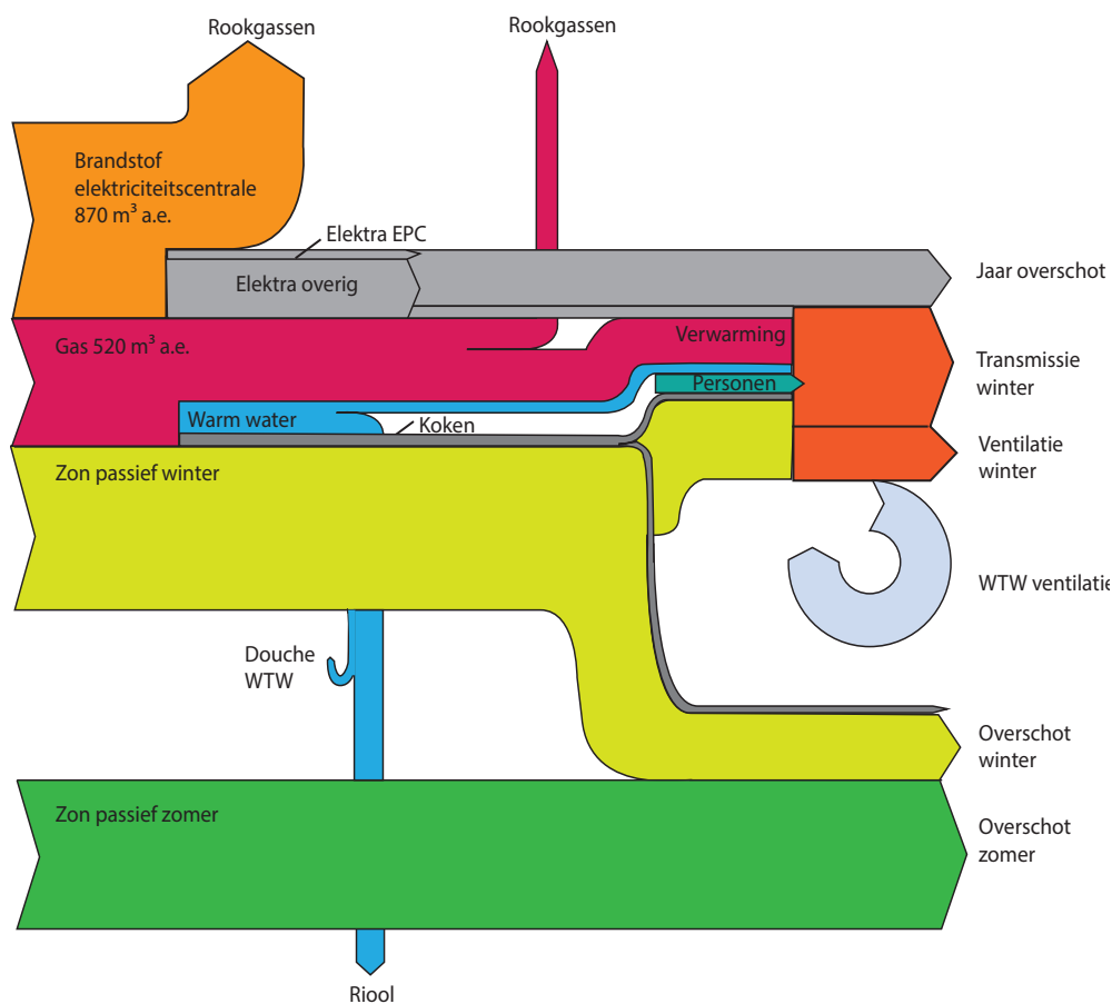
Afb. 1.14 Een indicatie van de energiestromen in de referentie tussenwoning (voorzien van pakket 1, zie paragraaf 3.4) voor een gemiddeld huishouden op basis van EPC-berekening en statistische gegevens (met name voor elektriciteitsverbruik voor huishoudelijke apparaten) in m 3 aardgasequivalent per jaar. Een dergelijk stromendiagram wordt wel een Sankey-diagram genoemd
