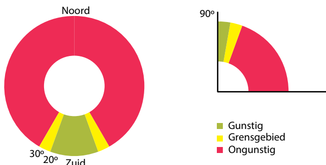
Afb. 4.15 Optimale oriëntatie en hellingshoek voor ramen. Een hellingshoek van 90° heeft de voorkeur om te hoge temperaturen in de zomer te voorkomen. Bovendien is de nachtelijke uitstraling bij verticale ramen het geringst. Als er houten kozijnen gebruikt worden, is het uit het oogpunt van onderhoud sowieso ongewenst om ze onder een hellingshoek aan te brengen
