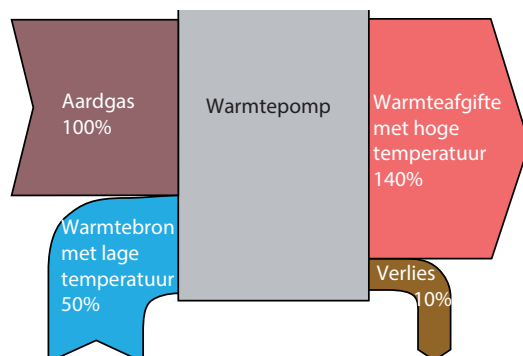
Afb. 7.24 Sankey-diagram van een gasgestookte warmtepomp
