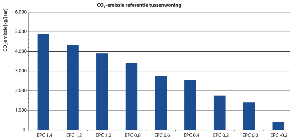
Afb. 2.2 De staafdiagrammen geven de CO 2 -emissie behorend bij het energieverbruik uit afbeelding 2.1
