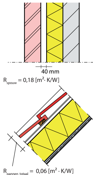
Afb. B.1-7 Warmteweerstand voor veel voorkomende luchtlagen in een spouwmuur en in een hellend dak met dakpannen, volgens NEN 1068:2012/C1:2014 [107]. Bij toepassing van een reflecterende folie op de isolatie aan de spouwzijde bedraagt de R_{spouw} 0,57 i.p.v. 0,18. Let op dat het effect van de folie niet dubbel geteld wordt: èn bij het isolatiemateriaal (inclusief folie) èn bij de spouw.
