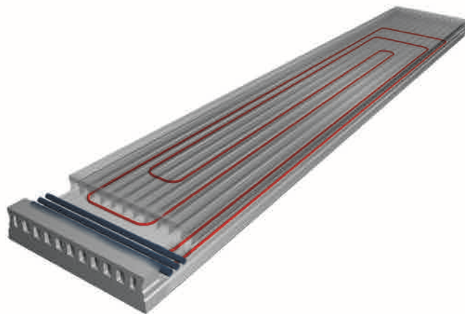
Afb. 7.7 Bij betonkernactivering wordt gebruik gemaakt van het accumulerende vermogen van de betonconstructies. De koel- en verwarmingsenergie wordt in de betonconstructie opgeslagen en wanneer nodig aan de ruimte afgegeven. 'Lage temperatuur verwarmen en hoge temperatuur koelen'. In woningen moet altijd ook een snel reagerend systeem aangebracht worden om aan de wisselende comfort eisen van de bewoners te voldoen. (Bron: VBI; prefab vloerelement met betonkernactivering)
