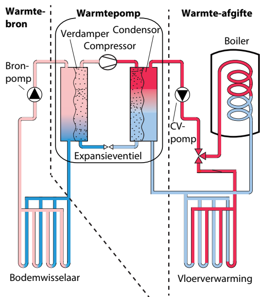
Afb. 7.21 Het principe van de warmtepomp
