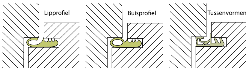
Afb. 0 Lipprofiel, Buisprofiel en Tussenvormen
