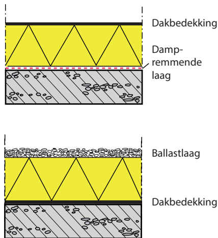
Afb. 5.12 Principe-opbouw van een warm dak en een omgekeerd (warm) dak. Bij het omgekeerde dak moet een ballastlaag worden toegepast tegen aantasting door UV-straling, wegwaaien en opdrijven van de isolatie; deze ballast kan bijvoorbeeld bestaan uit grind, een extensief vegetatiedak of tegels met tegel-dragers; bij fijner grind is een (dampopen!) folie nodig tussen grind en isolatie, maar dan kan wel de laagdikte van het grind geringer zijn ten opzichte van grof grind. Zeker bij een omgekeerd dak is een goed afschot gewenst. Meer informatie via www.sbrcur.net.nl : 'Infoblad 38: Een omgekeerd dak zonder waterplaten' en bij diverse fabrikanten
