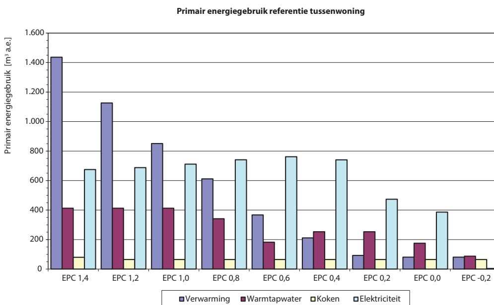
Afb. 2.1 De afbeelding geeft het primaire energieverbruik aan voor verwarmen, warmtapwater, koken en het huishoudelijke elektriciteitsverbruik (na aftrek van opbrengst PV) van de referentie tussenwoning (zie bijlage 4) met een EPC aflopend van 1,4 naar -0,2. Het verbruik voor ruimteverwarming en warmtapwater is berekend met NEN 5128:2004 voor de EPC's van 1,4 t/m 0,8 en met NEN 7120:2011 voor de EPC van 0,6 t/m -0,2. Het verbruik voor elektriciteit na aftrek van hulpenergie voor de installaties en koken is het gemiddelde verbruik per Nederlands huishouden (dus niet specifiek voor nieuwbouwwoningen) in respectievelijk 1996, 1998, 2000, 2006, 2011 en aanname voor 2015 op basis van 2012 (bron: Energie Trends 2014 [19]). Voor de EPC's 0,2 t/m -0,2 is gerekend met een kleine besparing op het huishoudelijk elektriciteitsverbruik. De EPC's van 0,2 t/m -0,2 zijn ter illustratie toegevoegd en zijn nog niet wettelijk vereist.
