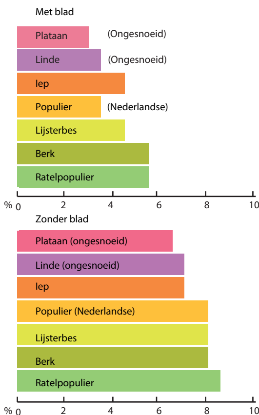
Afb. 4.10 De doorgelaten hoeveelheid zoninstraling in procenten t.o.v. de totale hoeveelheid opvallende zoninstraling. Zonder blad wordt 65 tot 85% van de op de bomen vallende zon doorgelaten. Een ratelpopulier laat dus de meeste zon door [78]
