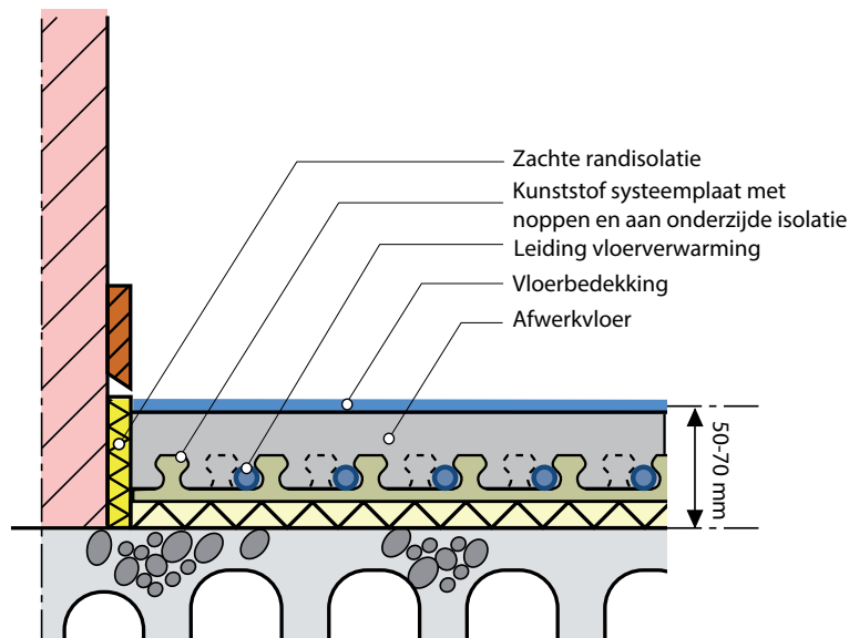
Afb. 7.6 Voorbeeld van de opbouw van een natbouwsysteem (zandcement of anhydriet) voor vloerverwarming. Voor een goede geluidsisolatie (als dat aan de orde is) moet onder en naast de zwevende dekvloer waterdichte (PE-)folie en een relatief zacht isolatiemateriaal gebruikt worden, bijvoorbeeld drukvaste minerale wol; hiervoor zijn specifieke producten verkrijgbaar. De folie voorkomt dat specie of anhydriet weglekt en daarmee mogelijk, na uitharding, de geluidsisolatie deels teniet doet. De plinten moeten vrij blijven van de dekvloer
