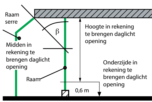
Afb. 4.23 De bepaling van de overstekhoek \beta van overstekken als gevolg van een overstek boven een serre.
