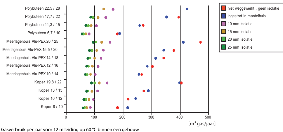
Afb. 9.7 Warmteverlies van leidingen bij verschillende isolatiediktes. Het is duidelijk dat een ribbelbuis of een kale kunststof leiding geen isolerende werking van betekenis heeft
