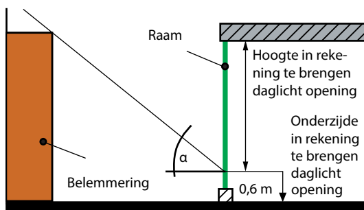
Afb. 4.21 De bepaling van de belemmeringshoek \alpha van belemmeringen binnen de perceelgrens. Alleen belemmeringen binnen een horizontale kijkhoek van 60° tellen mee.
