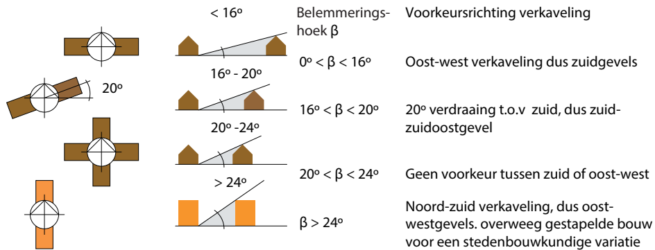
Afb. 4.4 Verkevelingsrichting voor eengezinswoningen bij een bepaalde belemmeringshoek
