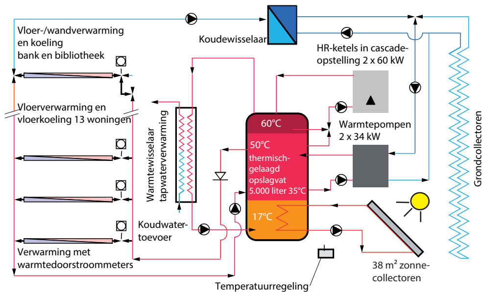
Afb. 7.23 Principeschema installatie voor verwarming en koeling van het voorbeeldproject Rabobank Pey-Posterholt in Echt te Limburg [171]. Het project omvat zowel een bank, een bibliotheek als dertien woningen. De installatie voor ruimte- en tapwaterverwarming (en koeling) is collectief. Twee warmtepompen onttrekken warmte uit de bodem of uit de vloerkoeling van de bank. De warmtepompen geven deze warmte af aan een opslagvat van 5 m 3 . Ook de zonnecollectoren (circa 40 m 2 ) geven hun warmte af aan dit (buffer)vat. Eventuele extra verwarmingscapaciteit kan geleverd worden door twee HR-ketels die ook de warmte leveren voor het naverwarmen van het tapwater. De bank en bibliotheek zijn voorzien van vloer en wandverwarming, de woningen van vloerverwarming. De vloer- en wandverwarming' worden ook gebruikt voor de afgifte van koude. Deze koude wordt onttrokken uit de bodem of is afkomstig van de warmtepomp (als deze warmte produceert). (Bron: Opdrachtgever: Rabobank; Architect: Architectenbureau Keulers, Schrijen Coonen te Echt/Geleen; Adviseur: Boom-Maastricht; Realisatie: 1999)
