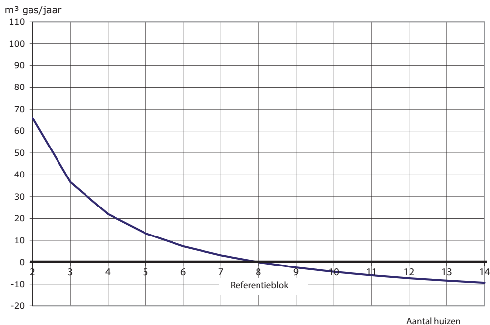
Afb. 4.2 De lengte van het bouwblok is van invloed op het gemiddelde energieverbruik voor ruimteverwarming per woning. Door de huidige goede warmte-isolatie is dit effect echter relatief beperkt. Door het verlengen van de bloklengte daalt het gemiddelde energieverbruik per woning; er komen immers meer tussenwoningen bij (met relatief weinig buitenoppervlak) terwijl het aantal kopwoningen gelijk blijft. Uitgangspunt bij deze afbeelding: de RVO-referentierijtjeswoningen (met pakket 1, zie paragraaf 3.4) voorzien van gebalanceerde ventilatie (systeem D3)
