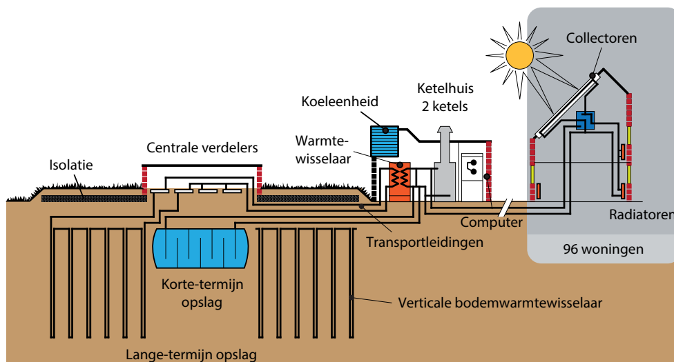
Afb. 7.34 Seizoenopslag voor zonnewarmte in het project Froukemaheerd in de Groningse wijk Beijum uit 1980. De opslag bestaat uit 15 km slangen aangebracht onder een centraal gelegen grasveldje. De opslag heeft een diameter van bijna 40 m en een diepte van 20 m en is aan de bovenzijde geïsoleerd. De 96 woningen zijn voorzien van totaal 2350 m 2 zonnecollectoren. Het verwarmingssysteem in de woningen bestaat uit lage temperatuur radiatoren. Er is een centrale bijstook met gasketels. Uit metingen blijkt dat de bijdrage van de zonne-energie aan de totale warmtevraag voor ruimte- en tapwaterverwarming ongeveer 65% bedraagt. De gemiddelde temperatuur van de bodem in de opslag varieert van circa 30 °C rond februari tot bijna 50 °C rond oktober. Het totale systeem functioneert nog steeds zonder bijzondere klachten. In de loop van de jaren zijn wel enige wijzigingen aangebracht en reparaties verricht [173]. In 2009 is het installatiesysteem gerenoveerd en aangepast [181]. Zo zijn er o.a. efficiëntere zonnecollectoren aangebracht zodat de collectoroppervlakte kleiner kon zijn en er ruimte vrij kwam om PV-panelen te plaatsen. De gewonnen warmte wordt nu (in tegenstelling tot voor de renovatie) direct in de desbetreffende woning voor tapwater gebruikt. Een overschot wordt per woonblok verzameld en voor ruimteverwarming gebruikt. Alleen als daarna nog warmte over is, wordt deze centraal opgeslagen. (Bron:
