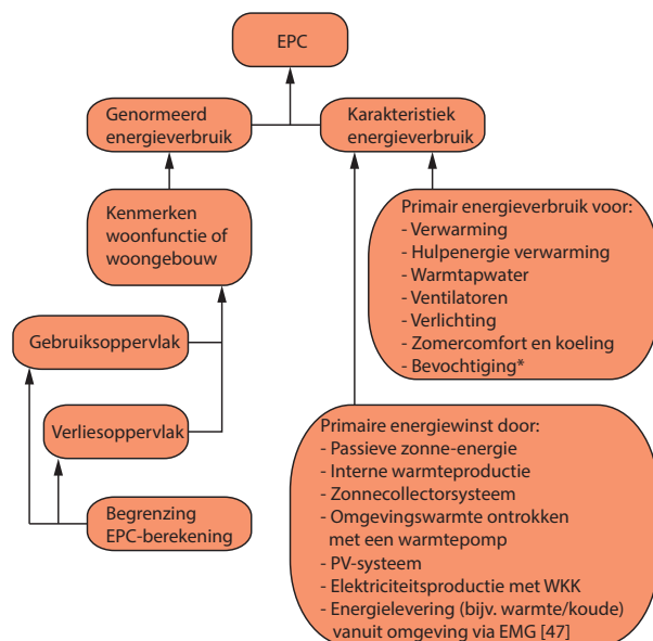
Afb. 2.5 Opbouw van de EPC; alle energieposten (op bovenwaarde) betreffen primaire energie per jaar
