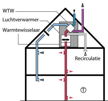
Afb. 7.10 Principe luchtverwarmingssysteem. De afstand tussen inblaaspunt en een gevel mag maximaal zo'n 6 meter bedragen
