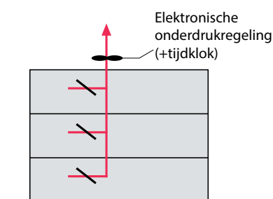
Afb. 6.17 Principe voor collectief systeem met een collectieve ventilator plus onderdrukregeling en kleppen per woning
