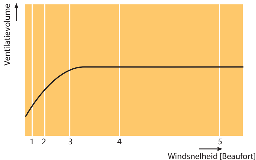
Afb. 6.10 Principe zelfregelend mechanisch ventilatierooster
