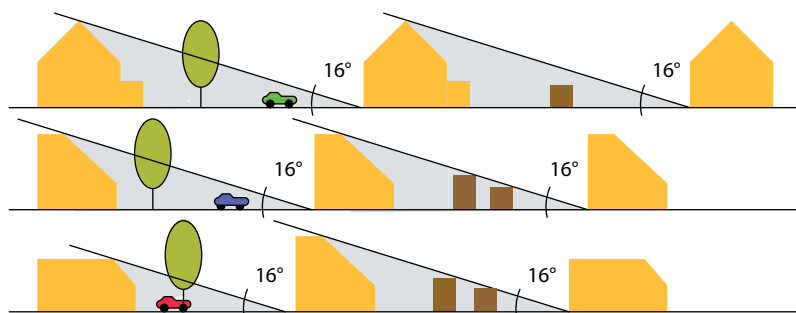
Afb. 4.9 Door verandering van de kapvorm en/of bouwvolume wijzigt de straatbreedte die nodig is om de belemmeringshoek tot 16^\circ te beperken [78]
