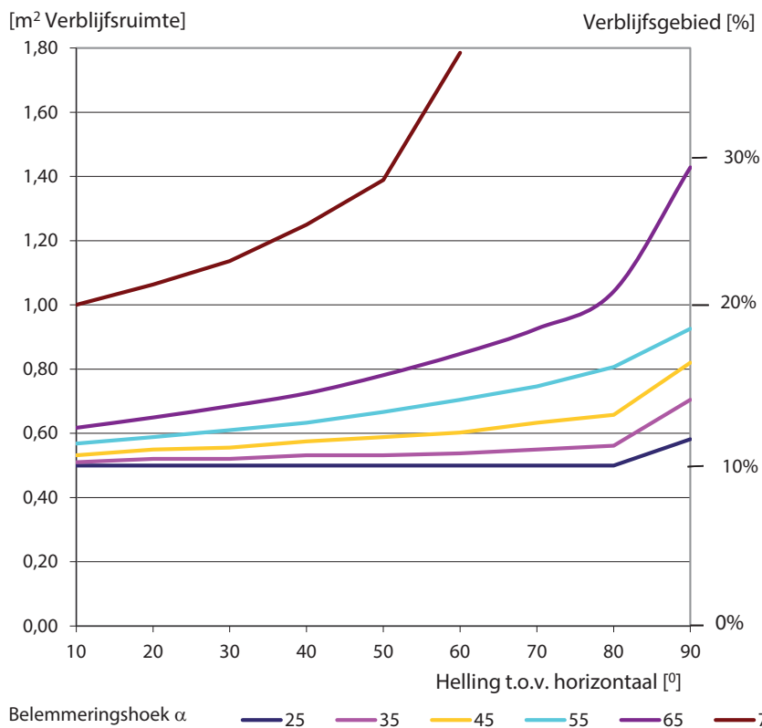
Afb. 4.25 Werkelijke daglichtopening om te voldoen aan de vereiste equivalente daglichtopening voor een dakraam voor een verblijfsruimte (links m 2 ) en verblijfsgebied (rechts %) bij verschillende belemmeringshoeken \alpha . De overstekhoek \beta is in alle gevallen 0. In alle gevallen ligt het hart van het raam op een hoogte van 1,7 meter. Berekend volgens NEN 2057 [82].
