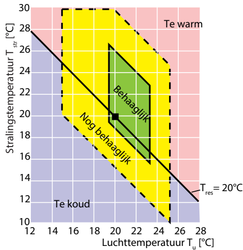
Afb. B.1-2 Samenhang tussen luchttemperatuur en stralingstemperatuur bij een relatieve vochtigheid van 30 tot 70% en een luchtbeweging van 0,1 tot 0,2 m/s. Uit de grafiek blijkt dat een T_{res} van 20 °C nog geen garantie hoeft te zijn voor een behaaglijk binnenklimaat. (Bron: [244])
