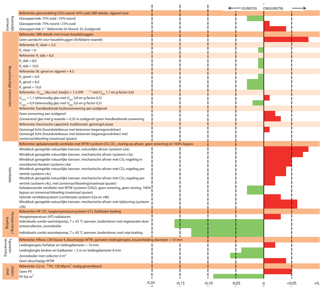
Afb. 3.2 Het effect van een aantal energiebesparende maatregelen op de EPC van de referentie twee-onder-een-kapwoning van RVO (voorzien van pakket 1 uit afb 3.3; EPC = ca. 0,4). De referentie-kenmerken staan in de horizontale grijze balken vermeld. Links in de gekleurde verticale balken staan de betreffende hoofdstukken. De EPC-effecten zijn afgerond op 0,01
