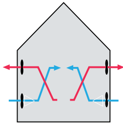
Afb. 6.19 Principe decentrale gebalanceerde ventilatie met WTW
