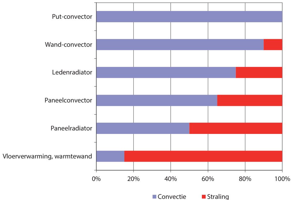
Afb. 7.2 Aandeel straling en convectie van de verschillende typen water-CV verwarmingselementen. Om eenzelfde gevoelstemperatuur te realiseren kan, bij een groter stralingsaandeel, de gemiddelde luchttemperatuur in een vertrek lager zijn. Dit werkt energiebesparend: Zowel de transmissie- als de ventilatieverliezen nemen af. Gebruik bij voorkeur een relatief lage watertemperatuur in combinatie met een relatief groot verwarmend oppervlak
