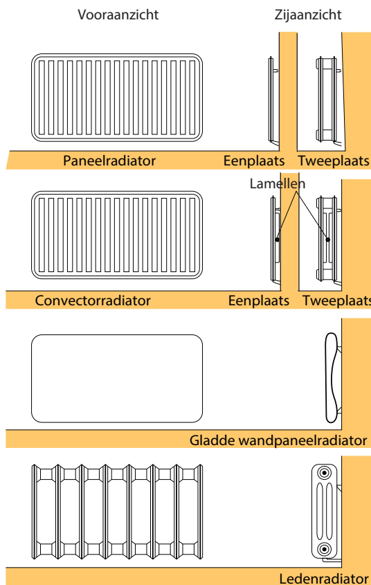
Afb. 7.3 De verschillende typen radiatoren
