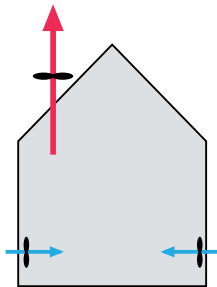
Afb. 6.20 Principe gebalanceerde ventilatie met decentrale toevoer en centrale afvoer
