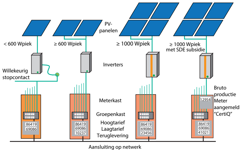
Afb. 10.3 Schematische weergave van mogelijkheden voor aansluiting op het openbare elektriciteitsnet
