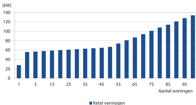
Afb. 9.12 Ketelvermogen voor een collectief systeem bij een buffer van 10 liter/woning bij CW4 [196].
