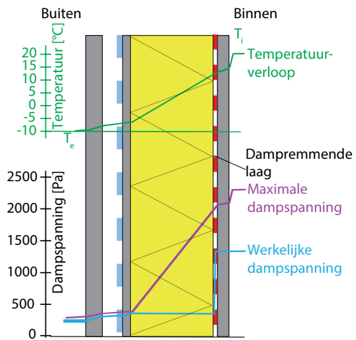
Afb. B.1-10 Een constructie moet van binnen naar buiten altijd een afnemende dampdichtheid hebben, anders kunnen er condensatieproblemen ontstaan. Een dampremmende laag moet daarom altijd aan de binnenzijde (woningzijde) van een constructie aangebracht worden, zoals in deze houtskeletbouw-constructie.
