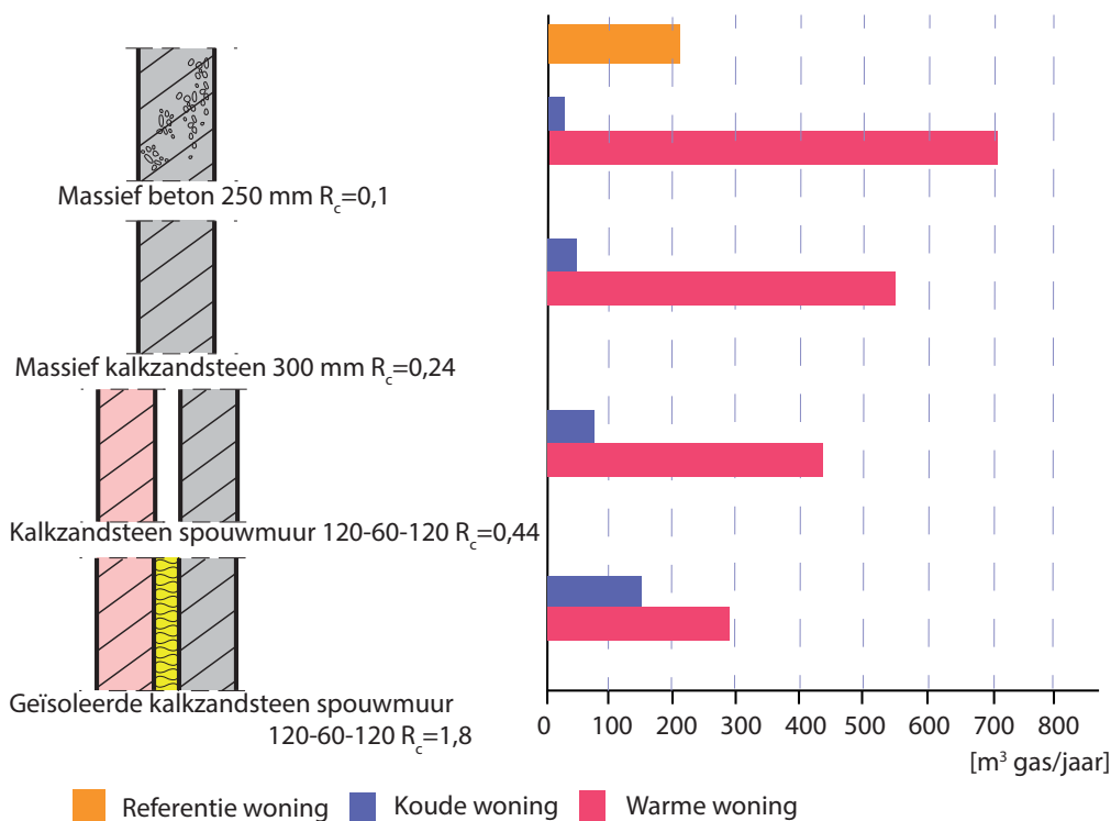
Afb. 5.25 Het energieverbruik in m^3 aardgas per jaar van de referentie tussenwoning wanneer hier gedurende het stookseizoen gemiddeld 2^\circ C meer (warme woning) of minder (koude woning) wordt gestookt dan in één van de aangrenzende woningen. Er is dus maar één woningscheidende wand met een temperatuurverschil van 2^\circ C . Het verbruik is afhankelijk van de isolatiewaarden van de woningscheidende wanden. De oranje balk geeft het energieverbruik van de referentiewoning aan als beide buurwoningen dezelfde temperatuur aanhouden als de referentiewoning. De spouwisolatie moet vanwege geluidisolatie uit een zacht materiaal bestaan, bijvoorbeeld onverpakte, minerale wol
