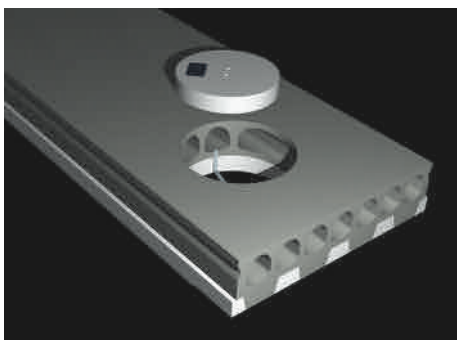
Afb. 5.9 Zorg er voor dat de isolatie onder een kruipluik goed aansluit op de isolatie van de vloer. Hiervoor bestaat een goede oplossing: een losse prefab isolatiedeksel dat in een speciale ophangbeugel geplaatst wordt. Kruipluik en isolatiedeksel zijn niet aan elkaar verbonden. Het hier getoonde vloerelement is voorzien van een door de fabrikant geboord kruipgat. Gebruik een goed luchtdicht kruipluik met een soepele
