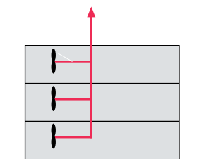
Afb. 6.16 Principe voor collectief systeem met individuele ventilatoren
