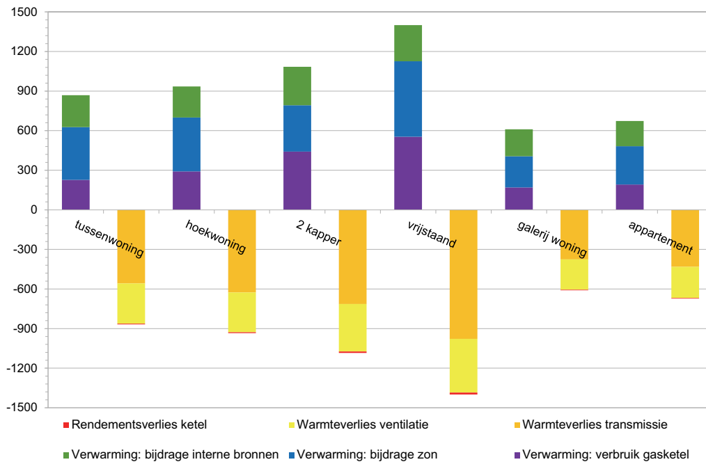
Afb. 1.13 De grafiek illustreert voor de zes RVO referentiewoningen met EPC van circa 0,4 (voorzien van pakket 1, zie paragraaf 3.4) de relevante warmtestromen voor ruimteverwarming (in m 3 aardgasequivalent)
