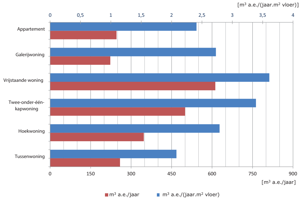
Afb. 4.1 De verschillen in het totale energieverbruik voor ruimteverwarming (gas + elektriciteit) plus elektriciteitsverbruik voor de ventilatie (in m³ aardgasequivalent per jaar) van de RVO-referentiewoningen (met pakket 1, zie paragraaf 3.4) met een EPC van circa 0,4 en voorzien van ventilatiesysteem D3 (gebalanceerde ventilatie met CO 2 -sturing op de afvoer). Het energieverbruik voor verwarming en ventilatie hangt af van grootte en compactheid van het woningtype. Om alleen het effect van compactheid te laten zien, is ook het energieverbruik per vierkante meter gebruiksoppervlak gegeven
