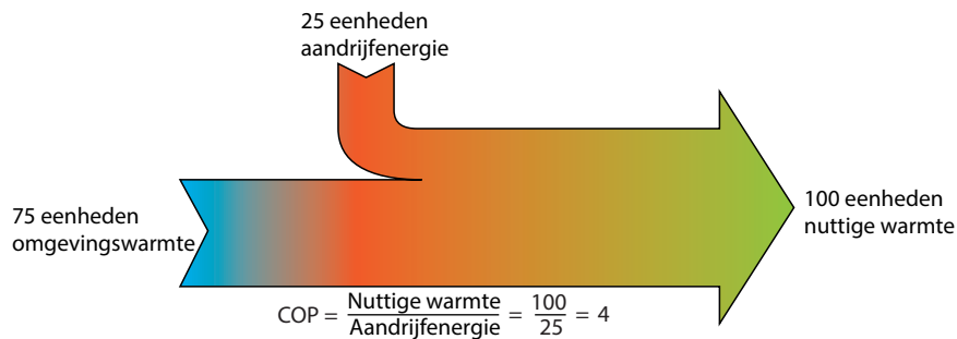
Afb. 7.20 De COP = 4. Dit betekent dat de warmtepomp 4 keer meer warmte (kWh thermisch) levert dan het apparaat als elektrische energie (kWh elektrisch) gebruikt. Naast 25% elektrische energie wordt 75% duurzame omgevingswarmte gebruikt bij verwarming van de woningen
