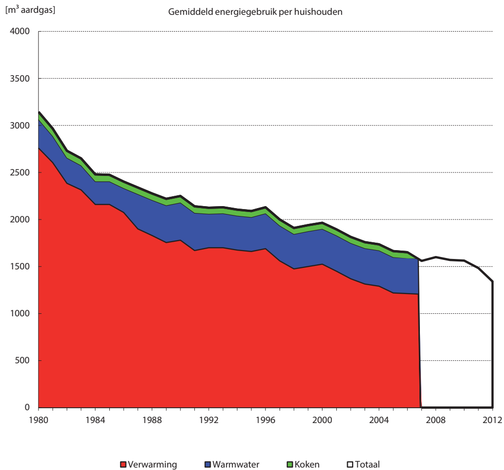
Afb. 1.9 Het gemiddelde aardgasverbruik voor verwarming, warmtapwater en koken per huishouden in de periode 1980-2012; (Bron: CBS met bewerking ECN en [19]. Vanaf 2008 is alleen het totale verbruik bekend)
