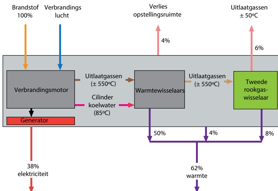
Afb. 7.28 Werkingsprincipe van een WKK-eenheid. Rendementen op onderwaarde
