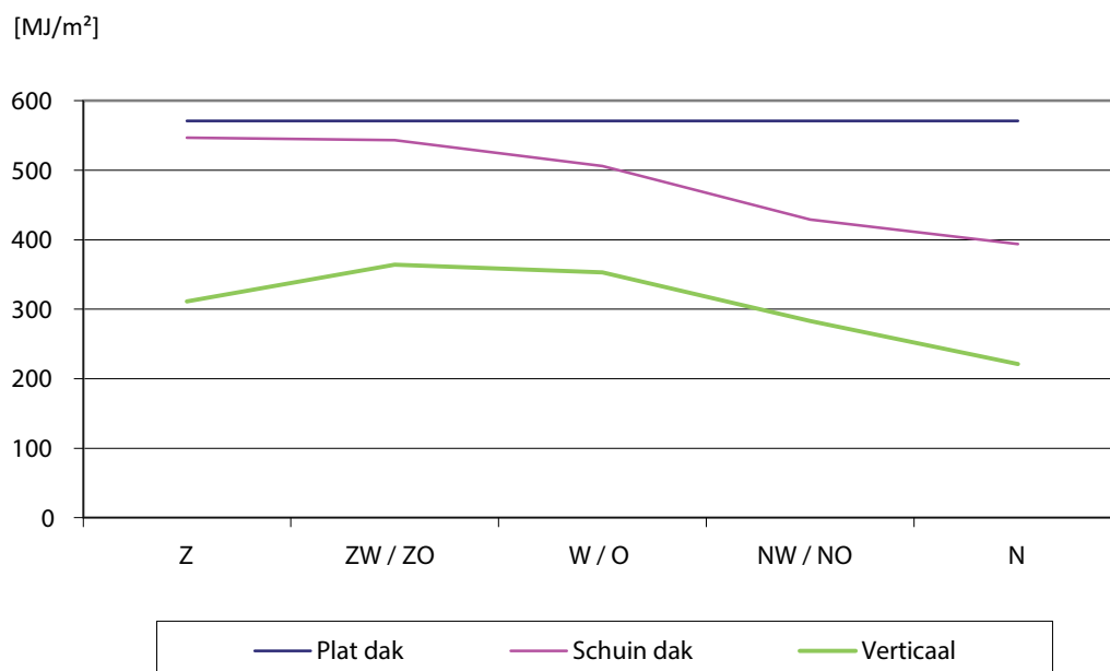
Afb. 4.14 De grafiek geeft de zonnestraling op een vierkante meter glas in de maand juni
