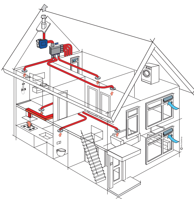
Afb. 6.14 Een variant op het standaard ventilatiesysteem C. Alle vertrekken zijn via luchtkanalen en een verzamel-luchtverdeelkast ('plenumbox') rechtstreeks aangesloten op de ventilatie-unit; in deze verdeelkast zitten één CO 2 - en één of twee luchtvochtigheidsensor(en), voor de badkamer(s), en een regelklep per vertrek. Deze kleppen worden door de sensor(en) aangestuurd waardoor elk vertrek optimaal geventileerd kan worden. (Bron: Itho Daalderop)
