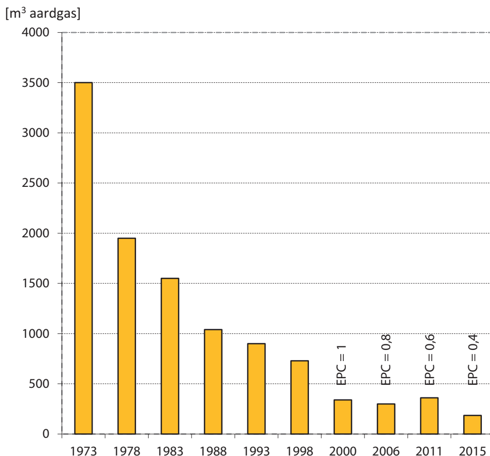
Afb. 1.10 Jaarlijks energieverbruik in m 3 aardgas voor ruimteverwarming (excl. elektriciteit voor CV-pomp) van een gemiddelde nieuwbouwwijteswoning gespecificeerd naar bouwjaar. Het gaat hierbij om berekende waarden. De waarden voor 2011 en 2015 zijn berekend met NEN 7120 (EPG). (Bron: [13] en referentiewoningen van RVO vanaf 1993)
