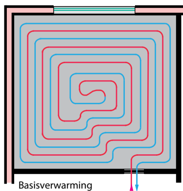
Afb. 7.8 Legpatronen vloerverwarmingsbuizen. Bij vloerverwarming als hoofdverwarming worden de leidingen bij de gevel vaak dichter bij elkaar gelegd (als compensatie van de 'koude' gevel) dan in de rest van de kamer
