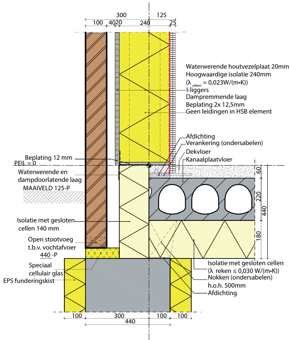
Afb. 3.8 Verticale doorsnede. Voorbeeld van de aansluiting fundering met langsgewel in een Passiefhuis. In het binnenspouwblad is een isolatiemateriaal gebruikt met een \lambda -waarde van 0,23 (bijv. PIR-schuim); als er minerale wol met een \lambda -waarde van 0,035 wordt gebruikt, neemt de isolatiedikte toe van 240 mm naar ca. 340 mm. Om de koudebrug van de constructie in het binnenblad te beperken is een houten I-ligger gebruikt. Het gemetselde buitenspouwblad staat op cellulair glas, eveneens om de koudebrug via de fundering te minimaliseren. Bron [63].
