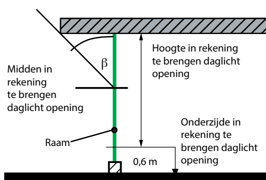
Afb. 4.22 De bepaling van de overstekhoek \beta van overstekken.
