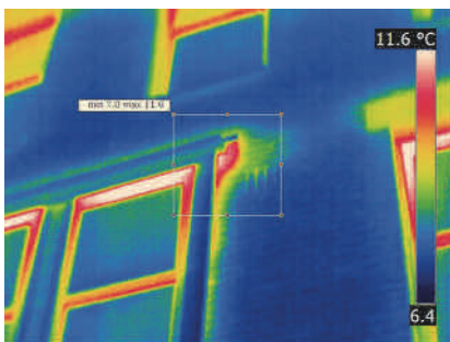
Afb. 5.1 Voorbeeld van een onderzoek door middel van thermografie. Duidelijk zichtbaar zijn de warmtelekken (als rode vlekken). (Bron: Nieman Raadgevende Ingenieurs)
