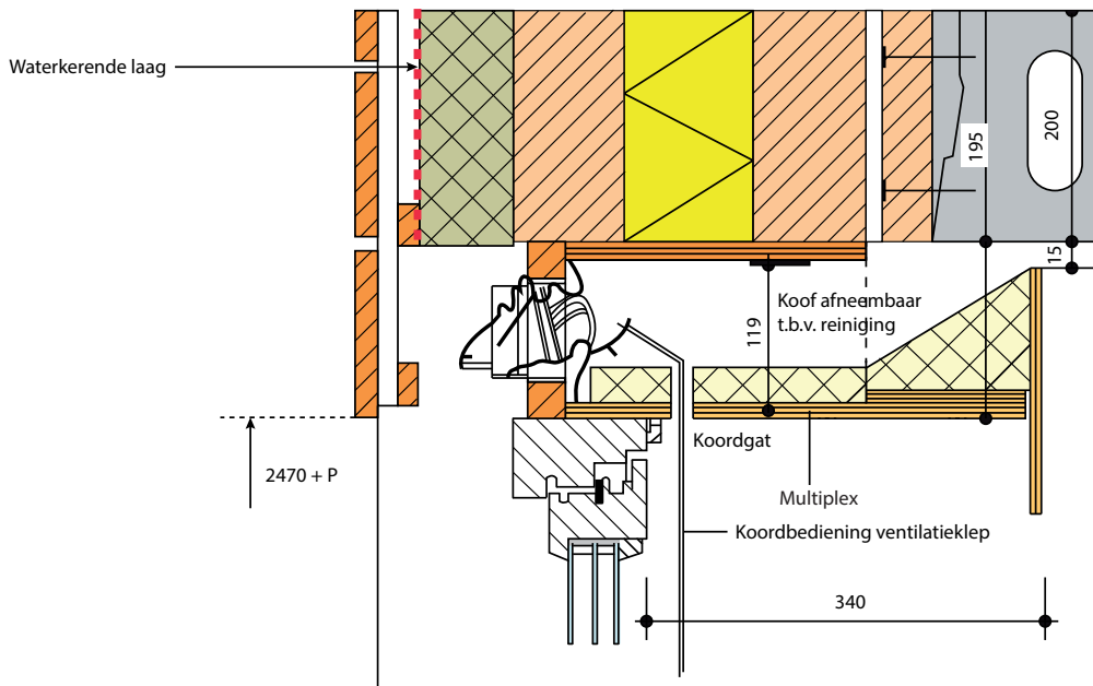
Afb. 6.12 Ventilatiooster met bouwkundige koof waardoor de binnenkomende luchtstroom langs het plafond wordt geleid; de 'uitmonding' (spleet) moet circa 15 mm hoog zijn om de lucht voldoende ver in het vertrek te leiden. De koof is te verwijderen ten behoeve van het schoonmaken van koof en ventilatiooster. Aan de onderzijde van de koof kunnen gordijnen worden opgehangen zodat die de toevoer van de ventilatielucht niet belemmeren. De koof is ontwikkeld voor de 'Brabantwoning' en in [134] toegelicht. (Bron: Renz Pijnenborgh, Archi Service)
