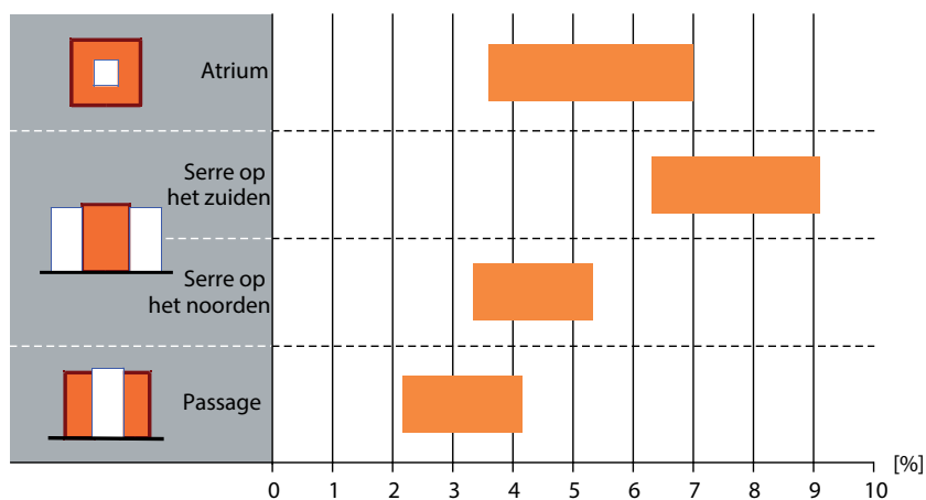
Afb. 4.19 Ventilatie zomersituatie. Globale indicatie van het gedeelte van de ventilatie-openingen (als functie van de vloeroppervlakte) dat benodigd is om de luchttemperatuur van de GGR minder dan 3 °C van de buitenluchttemperatuur te laten afwijken. De oppervlakte moet in principe zowel onderin als bovenin de GGR worden aangebracht (bron [81])
