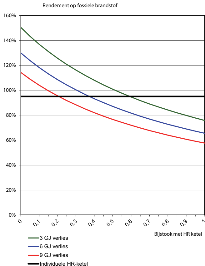
Afb. 7.36 Rendement op primaire energie van een collectief systeem afhankelijk van het percentage bijstook en het verlies van het distributiesysteem. 3 GJ verlies is alleen haalbaar bij blokverwarming, 9 GJ of meer is gebruikelijk bij warmtelevering. Uitgangspunten: rendement WKK 36% elektrisch, 50% warmte; rendement bijstook (HR-ketel op 75°C) 90%.; de warmtevraag (zonder bovenstaande verliezen) van de woning bedraagt 16 GJ inclusief tapwater. Rendement van de centrale opwekking die vermeden wordt is 50% conform NEN 7120 (zie in norm bij geëxporteerde energie). Alle rendementen op bovenwaarde. (Bron: BOOM-SI)
