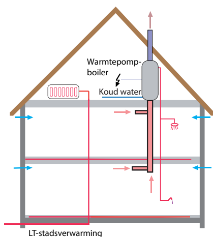
Afb. 9.23 Een schema van een warmtepompboiler
