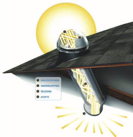
Afb. 4.20 Een 'daglichttub' of 'daklichtspot' kan handig zijn om een inpandig of diep vertrek van (meer) daglicht te voorzien als een dakraam of dakkoepel niet mogelijk is. De buis is inwendig voorzien van een zeer goed reflecterend materiaal. Er zijn diverse fabrikanten die dergelijke daglichtbuizen leveren. (Bron: Solatube International Inc.)
