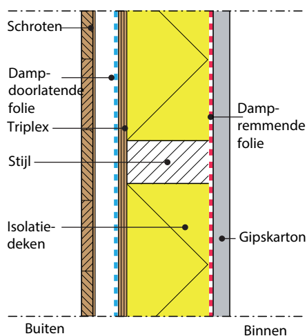
Afb. 5.24 Vooral bij houten gevel-elementen en houtskeletbouw is een dampremmende laag aan de binnenzijde (dus aan de warme zijde) vaak noodzakelijk. Zo'n laag is ook gunstig voor de luchtdichtheid van constructies
