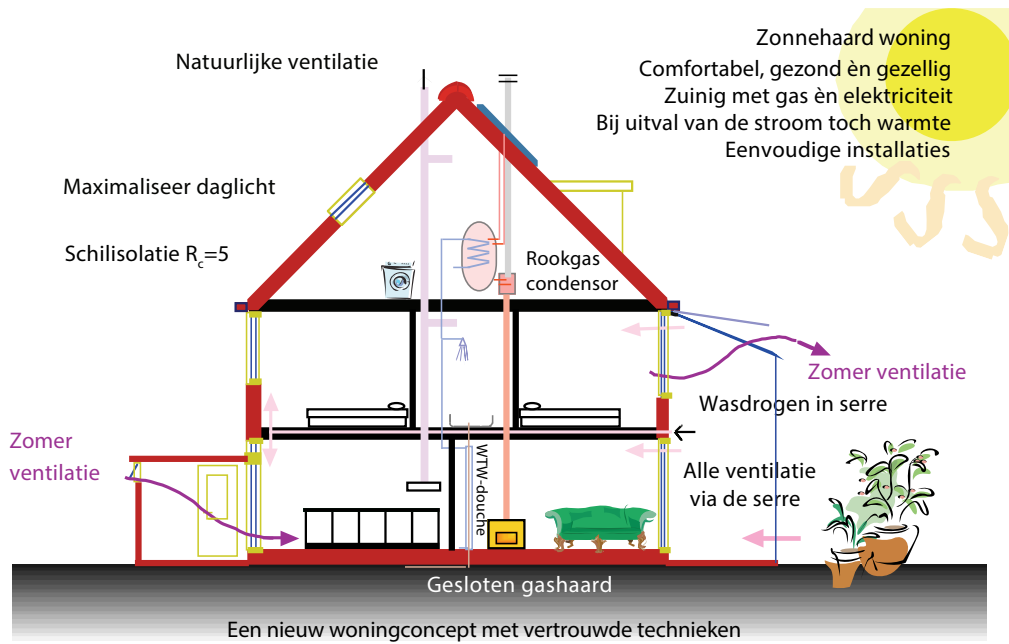
Afb. 3.10 Principe doorsnede van een zonnehaardwoning.
