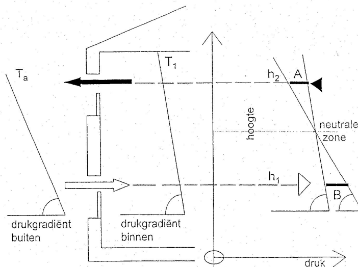
figuur 2. schematische weergave van het principe van thermische trek bij ventilatie-openingen die op verschillende hoogte in hetzelfde gevelvlak zijn gelegen
