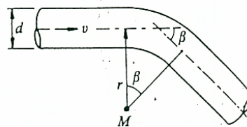
Bochtverliezen
