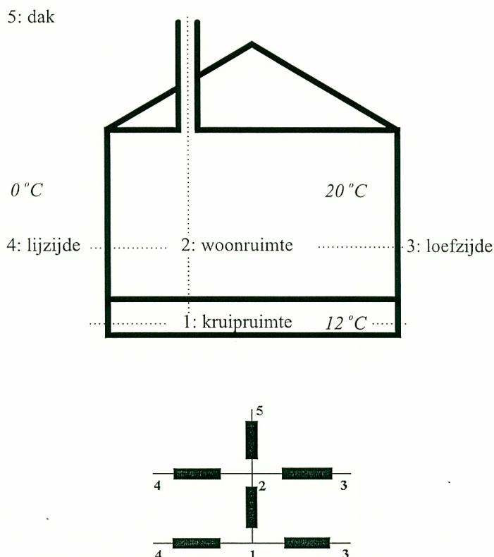
figuur 1. schematische doorsnede van een woning en het bijbehorende tweezone luchtstroommodel, weergegeven in een elektrisch analogon
